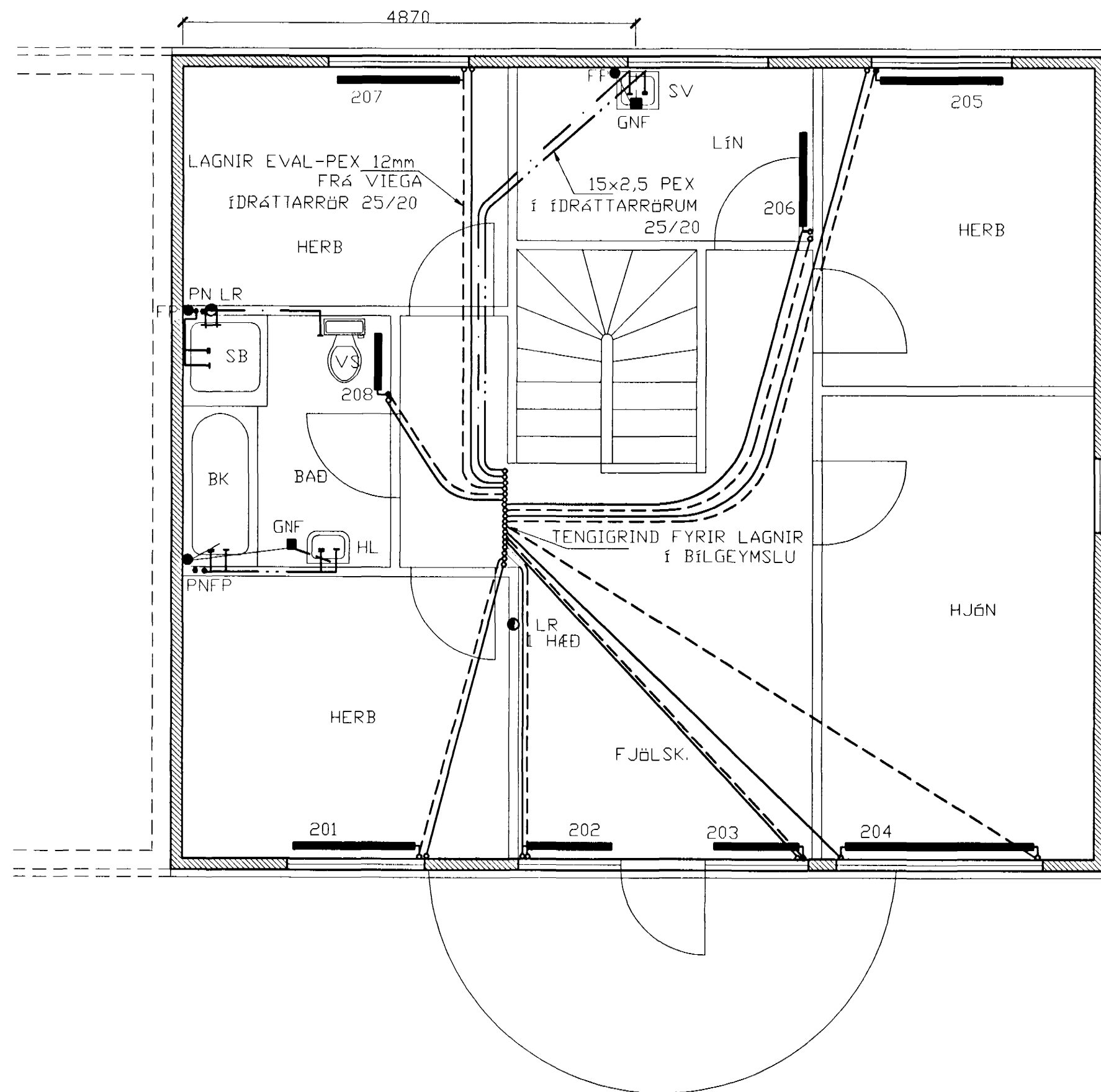
GRUNNMYND 2 HÆÐAR 1:50
