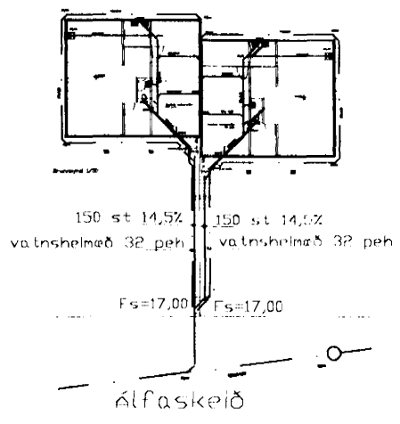
Afstöðumynd 1/500
