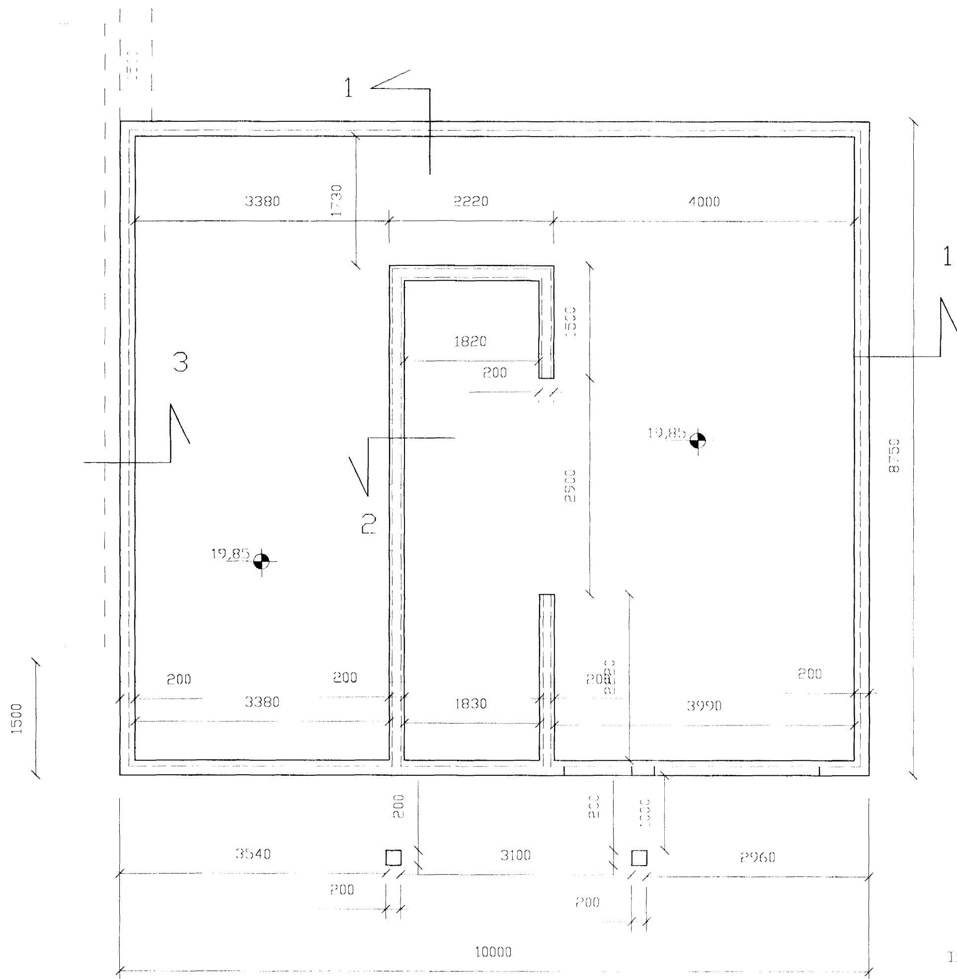
Grunnmynd 1/50
