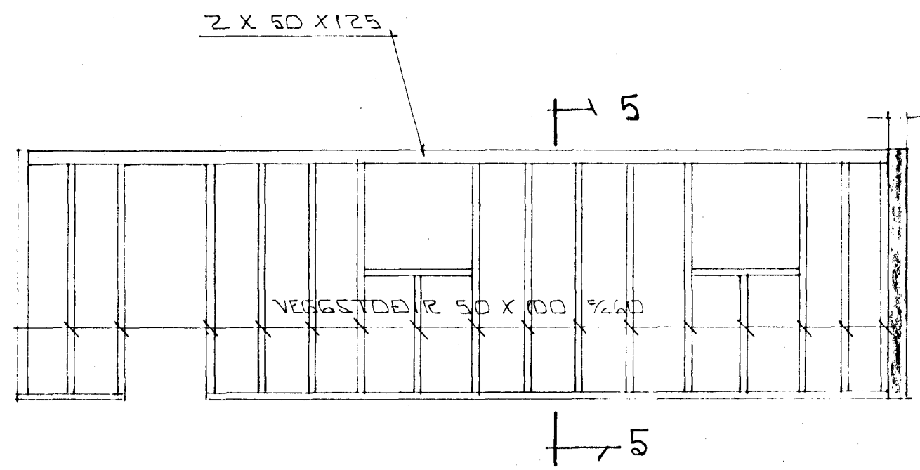
ÁSYND A - A ~ 1:50
