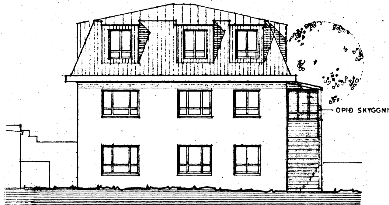
NORÐAUSTUR 1:100
