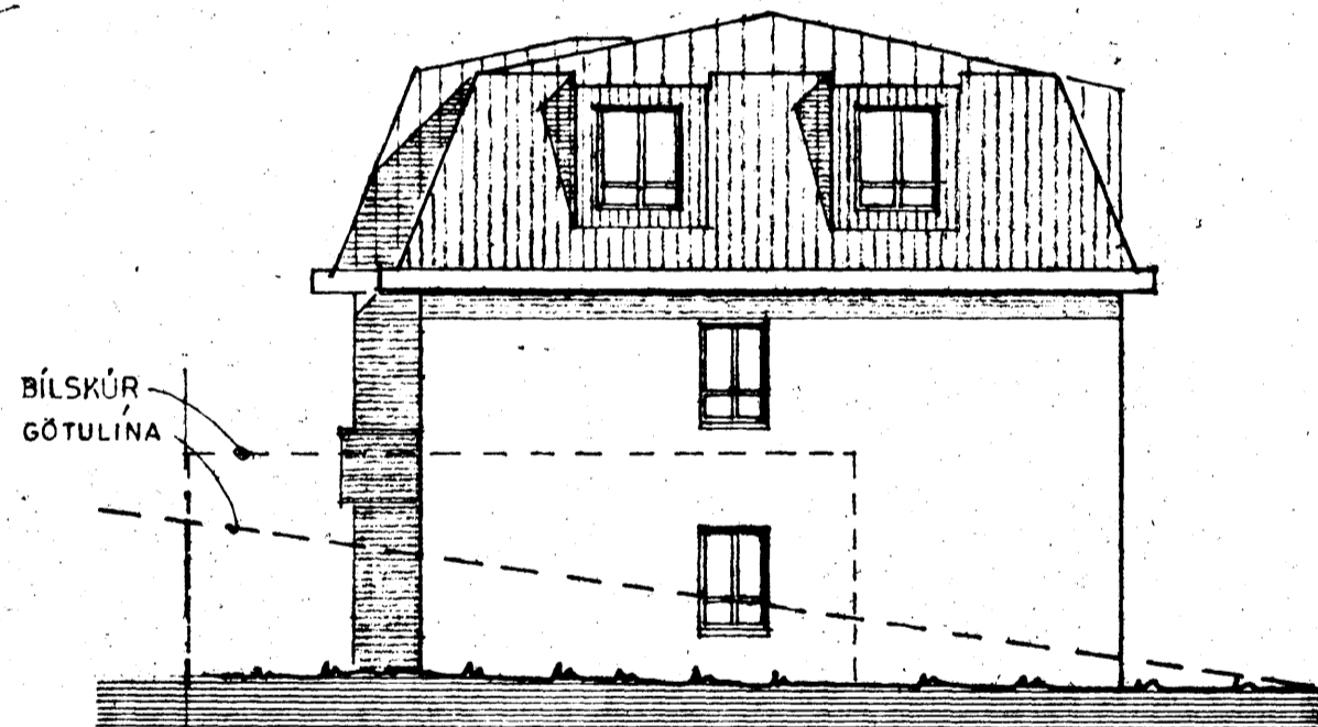
SUÐAUSTUR 1:100
