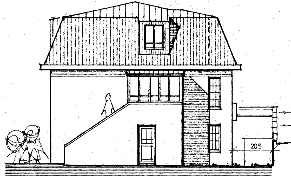
NORÐVESTUR 1:100
