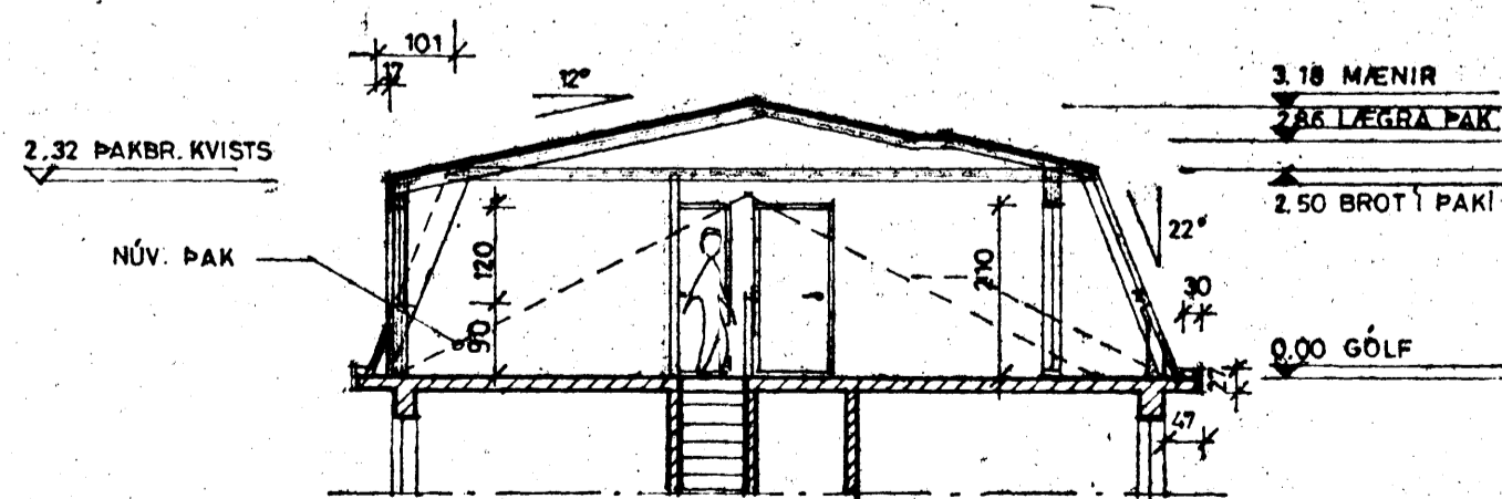
SNID 1:100 A-A
