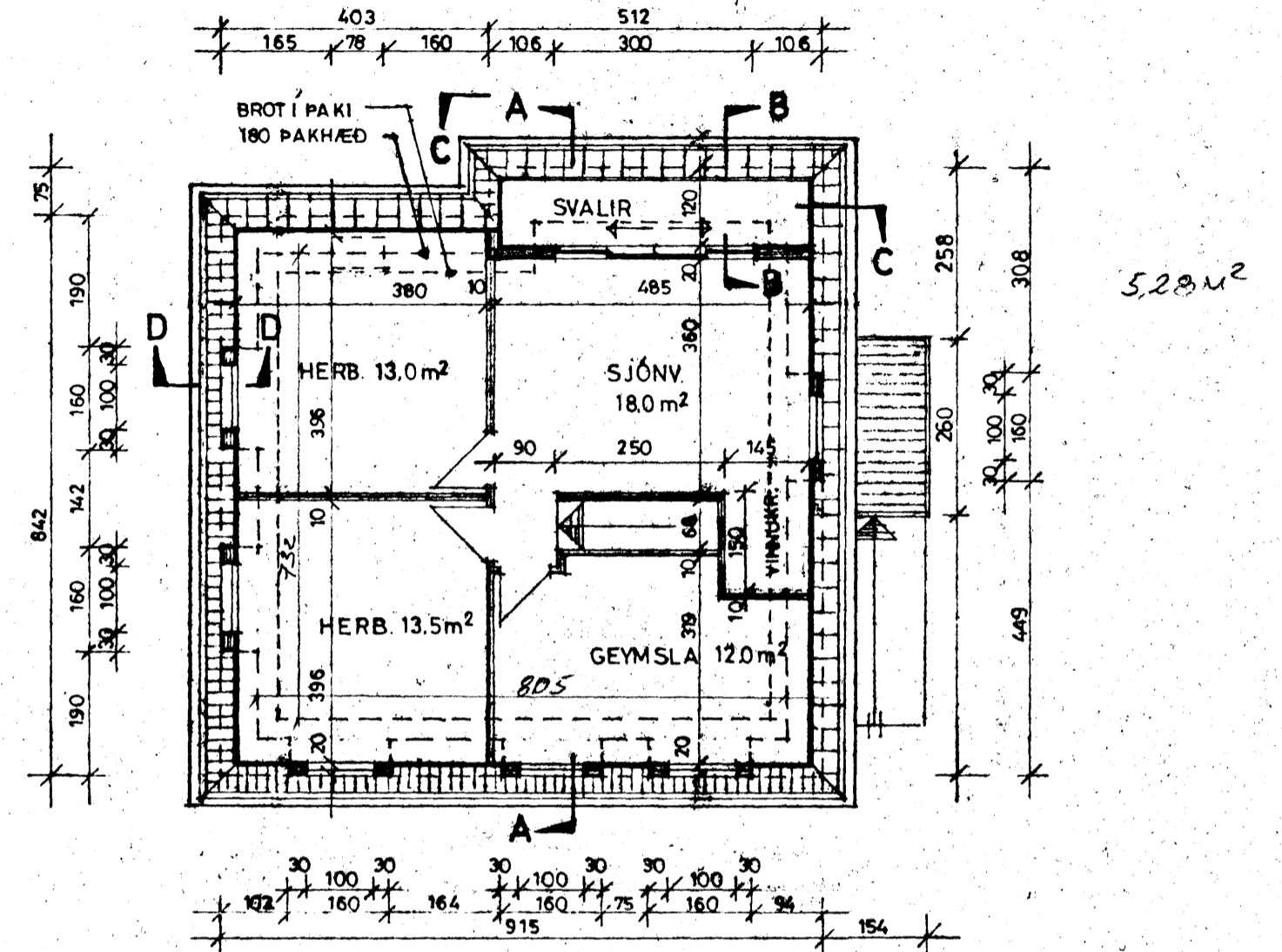
GRUNNMYND PAKHÆÐAR 1:100
