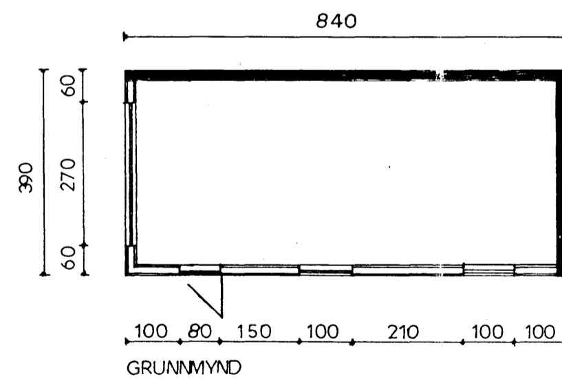
GRUNNMYND
