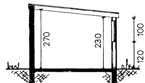
SNIÐ
