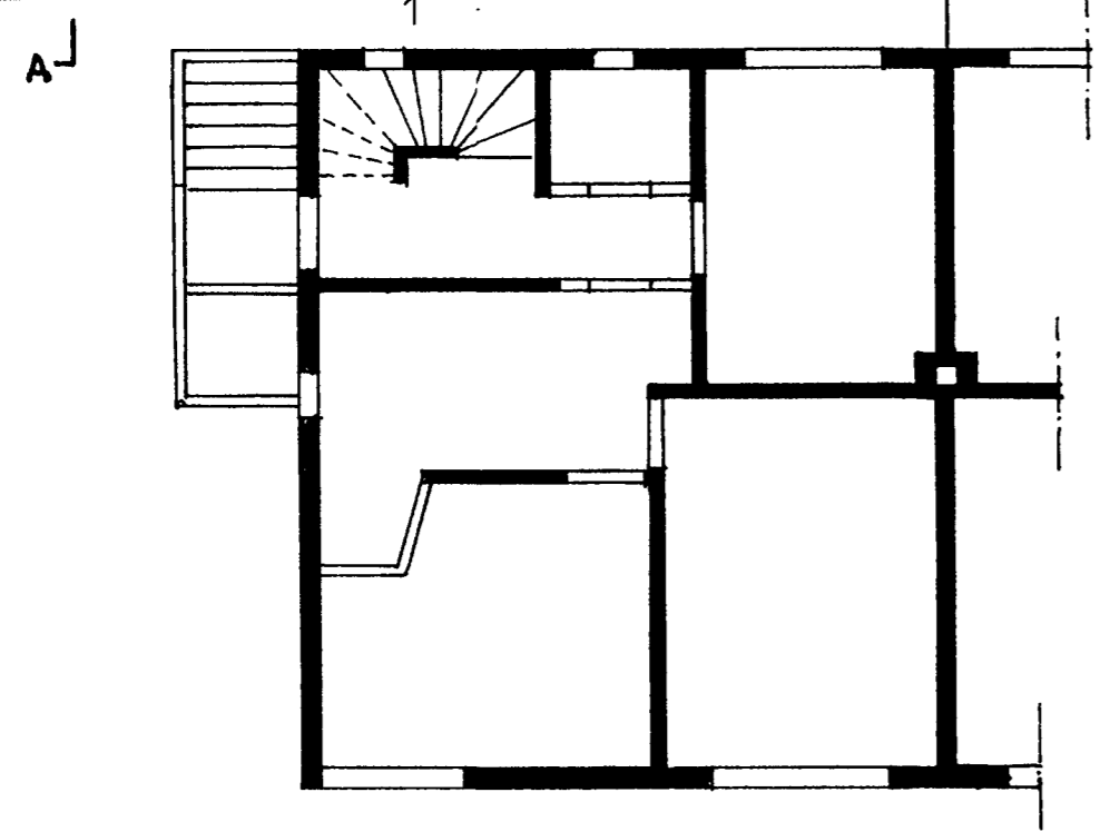
GRUNNMYND KJALLARA
