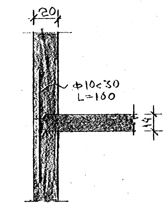
STEXPLUSKIL I UTVEGG -1:20-
