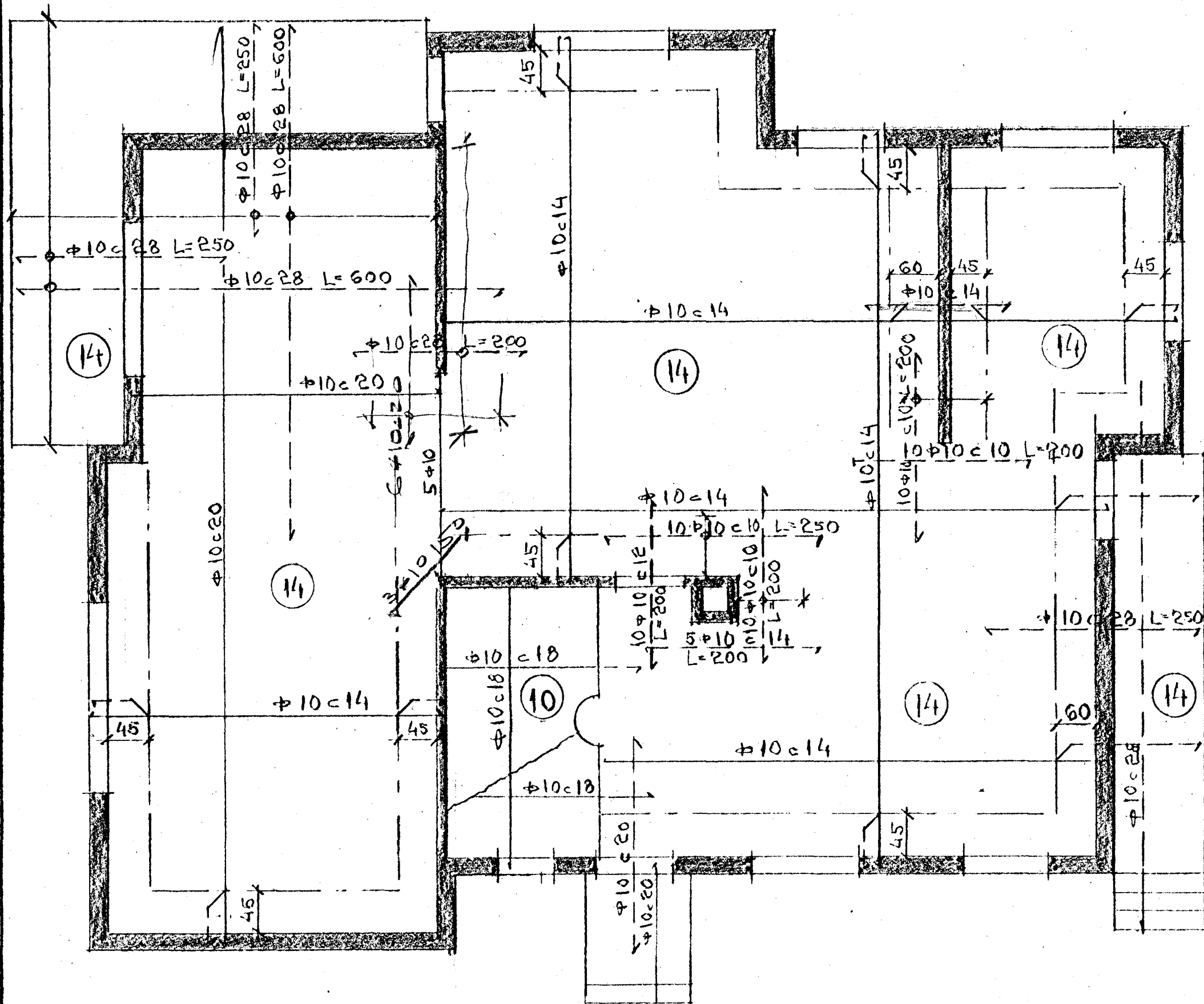
LOFT YFIR 1. HÆÐ 1:50 LOFT YFIR 2. HÆÐ ER EINS
