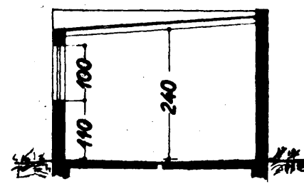
Snit A-A
