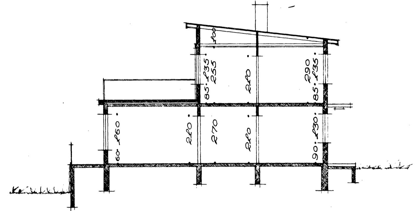
Sneiðing
