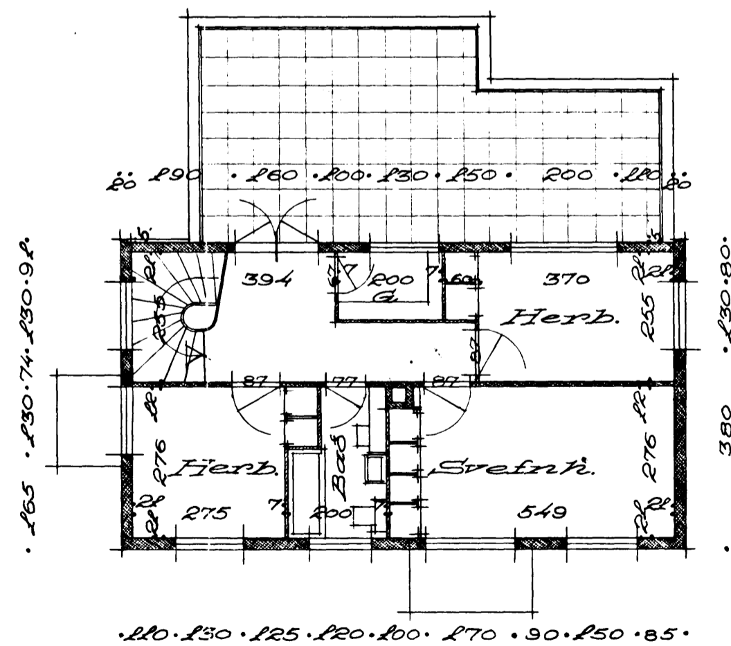
2. hæð
