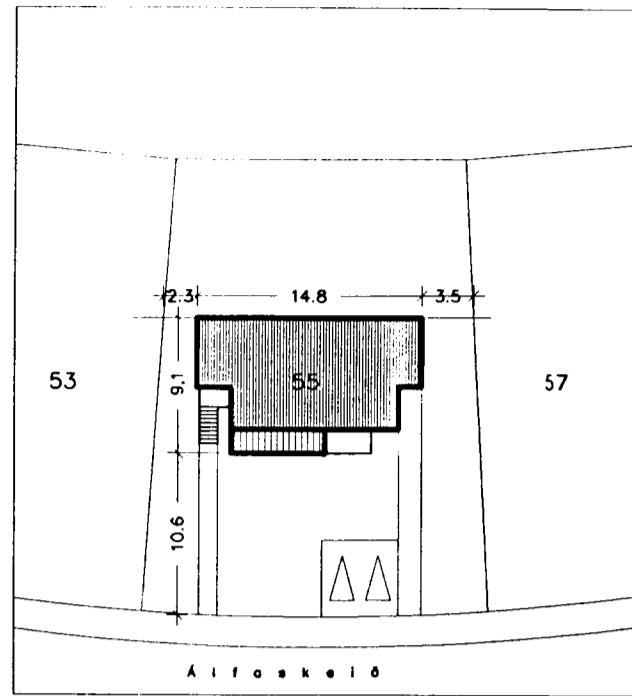
Afstöðumynd 1:500
