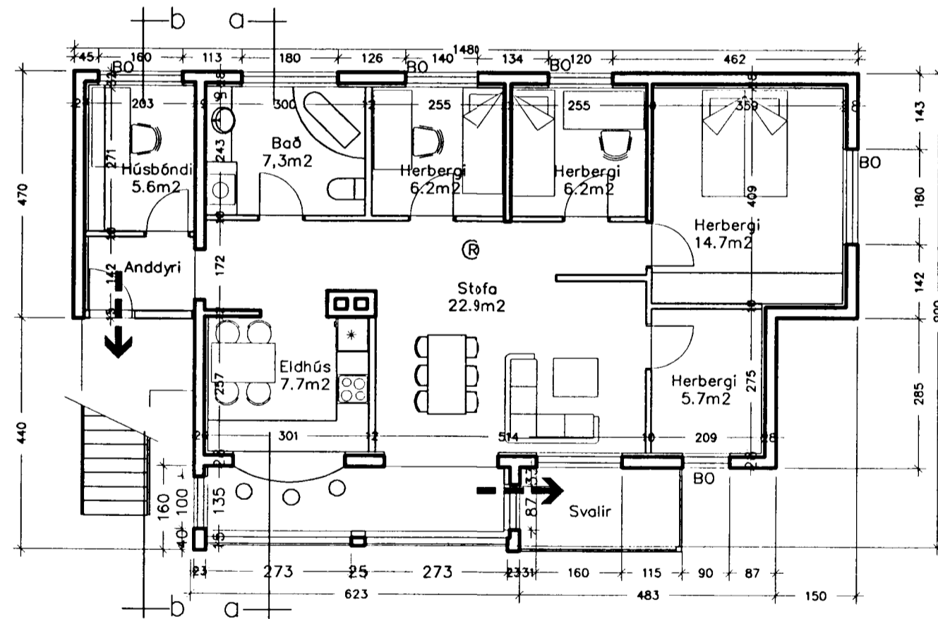
Grunnmynd 2.hæð 1:100
