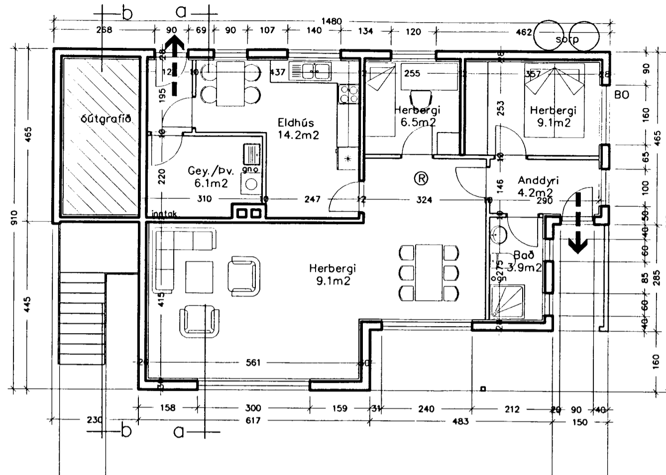
Grunnmynd 1.hæð 1:100
