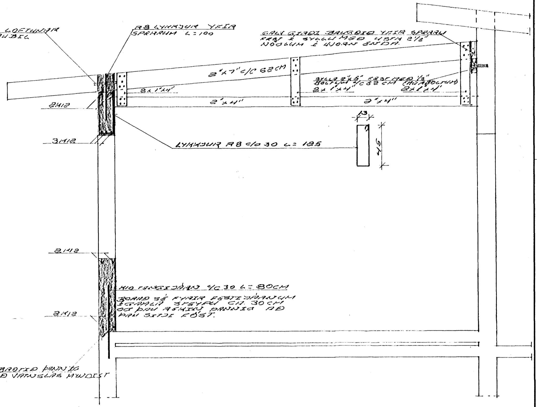
SNIÐ B-B M:1:80
