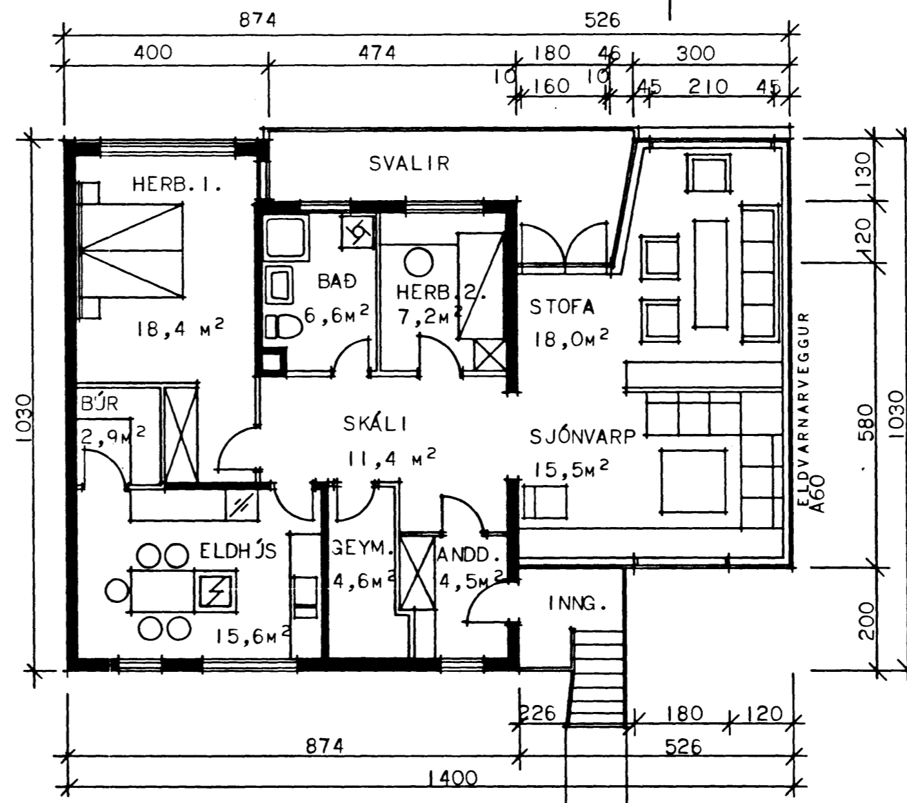
2. HÆÐ.
