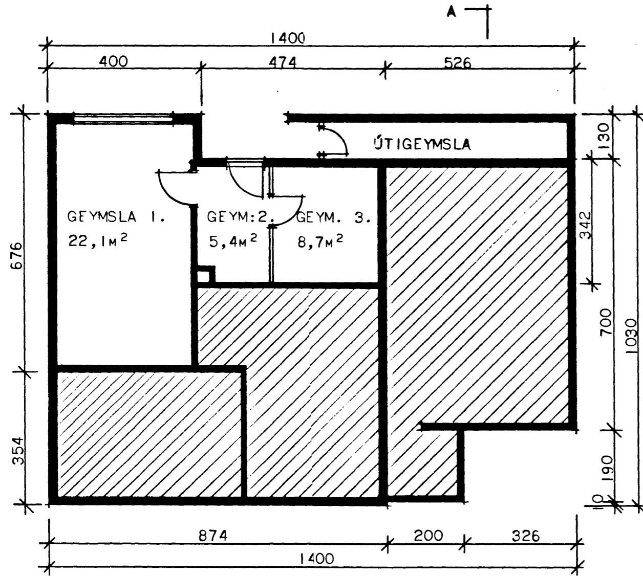
KJALLARI
