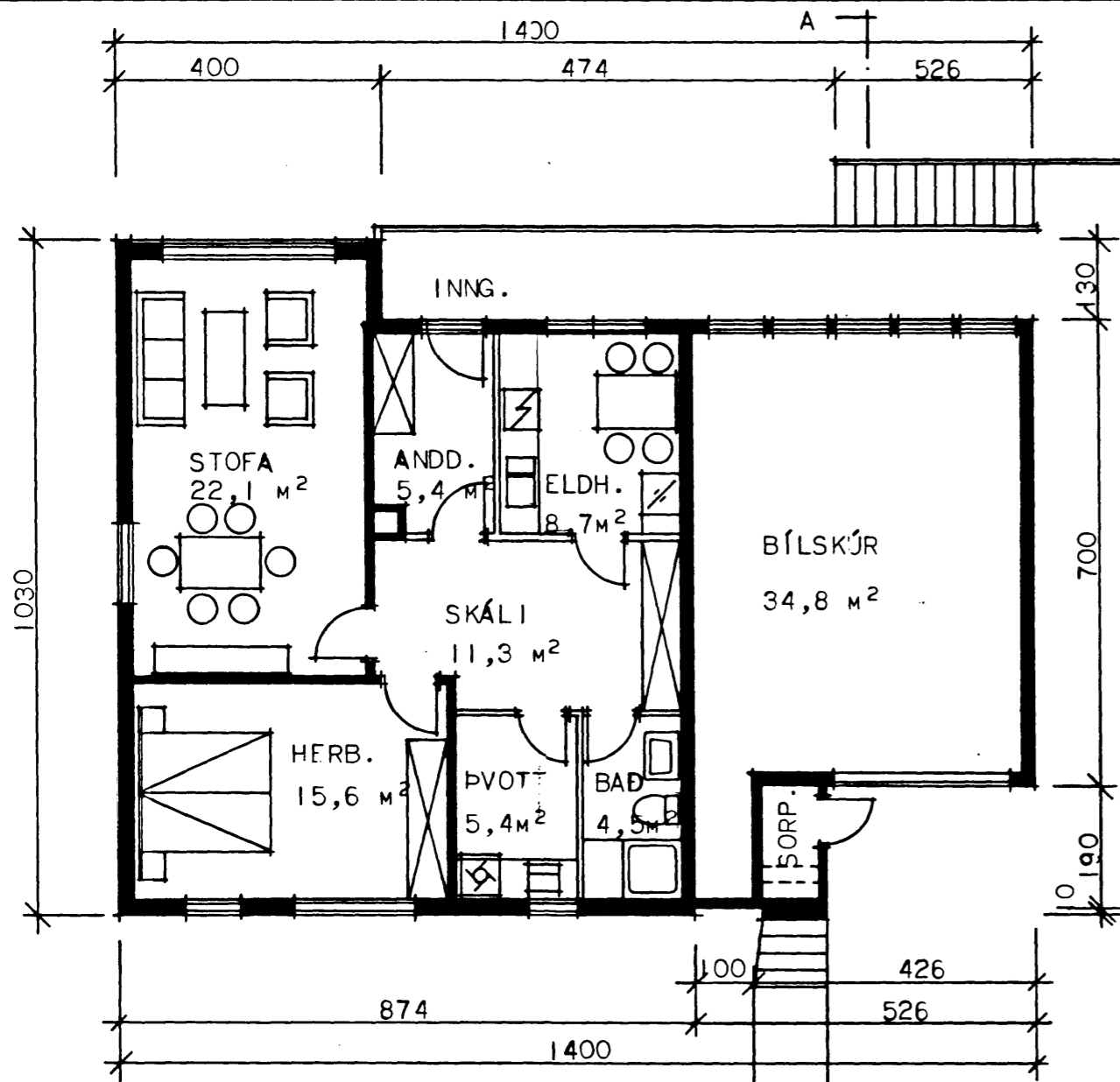
1. HÆÐ.
