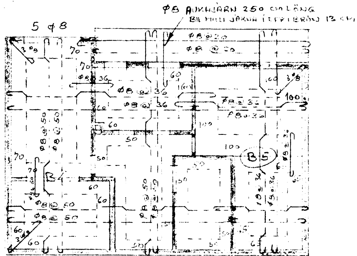
LOFT YFIR KJALLARA
