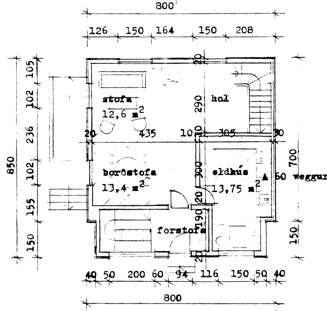
Grunnmynd 1. hæðar (jarðhæðar)
