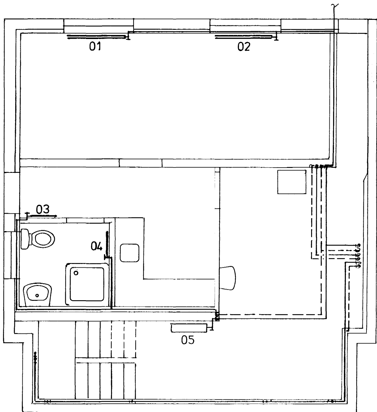
Grunnmynd kjallara
