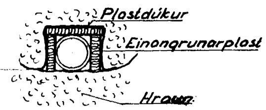
Einongrun frárennslíspípu 1:20
