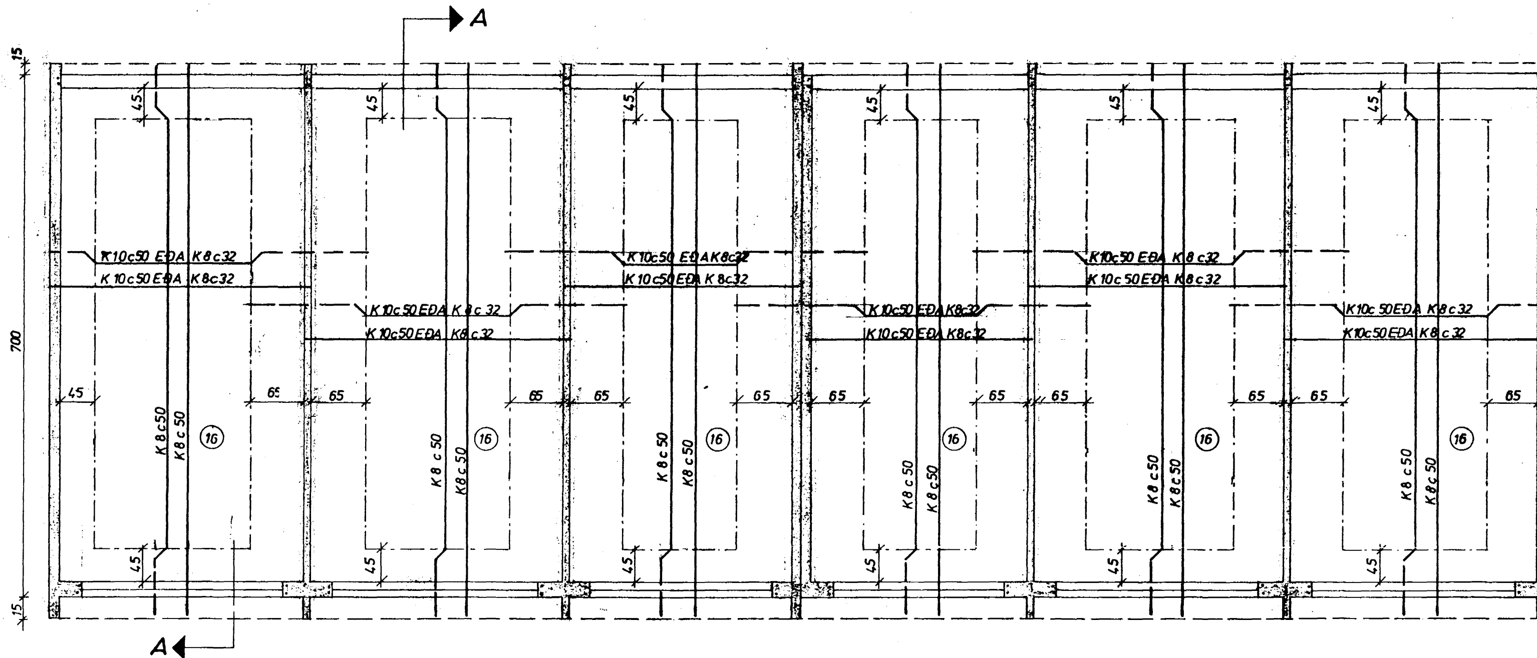
GRUNNMYND 1:50
