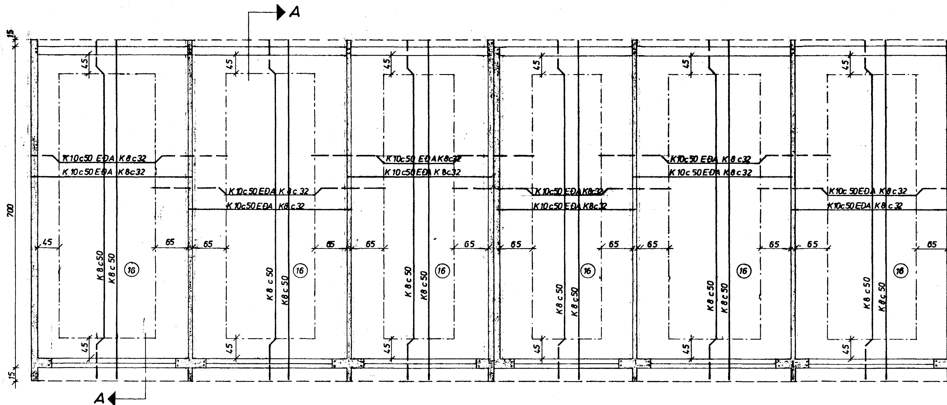
GRUNNMYND 1:50
