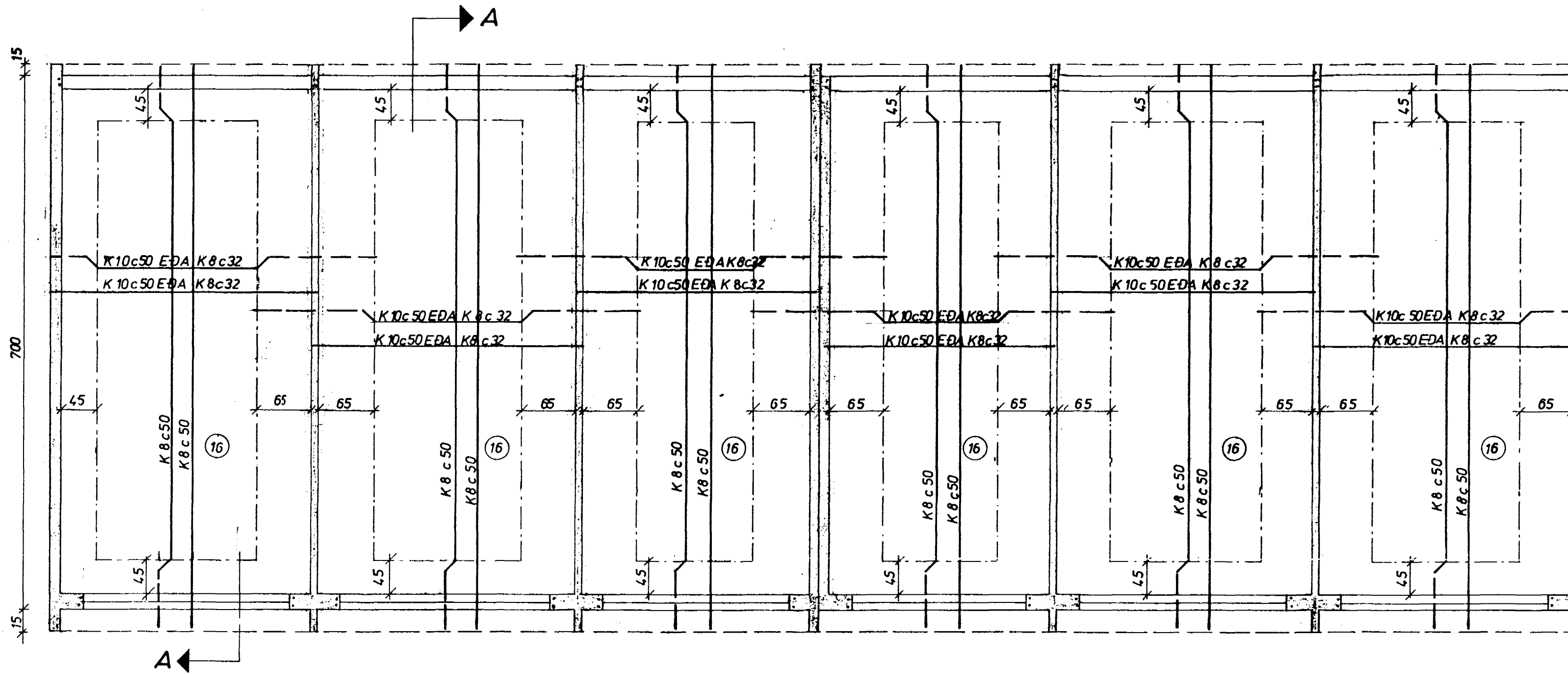
GRUNNMYND 1:50
