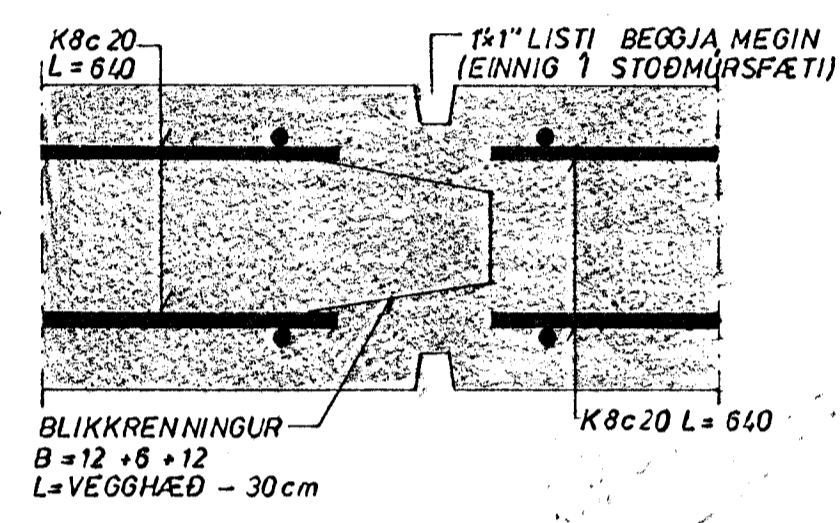
ÞANRAUF 1:5
