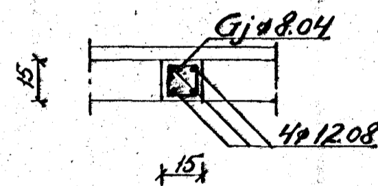
Snið B-B
