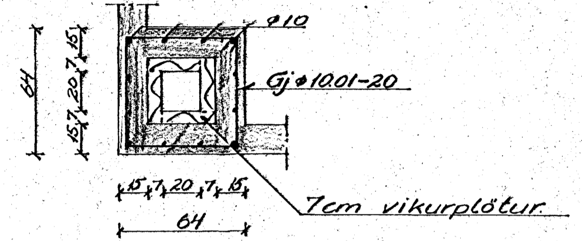
Reykhöfur 1:20
