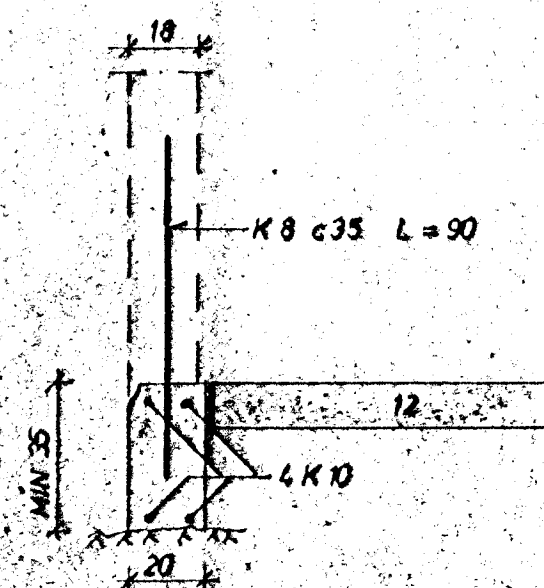
SNIÐ A 1:20
