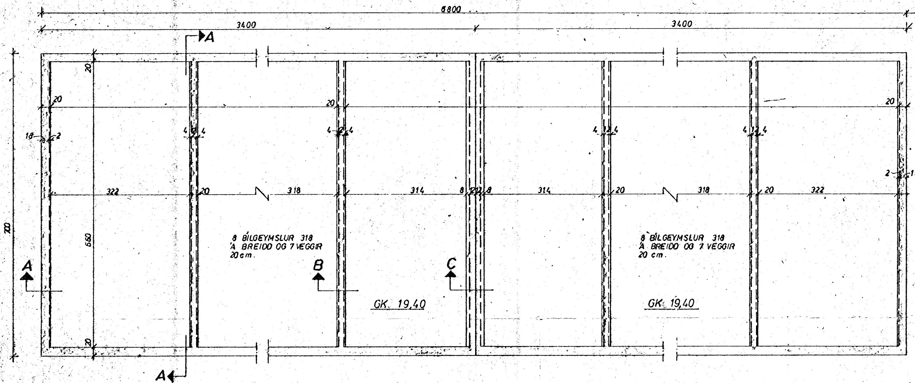
GRUNNMYND 1:50
