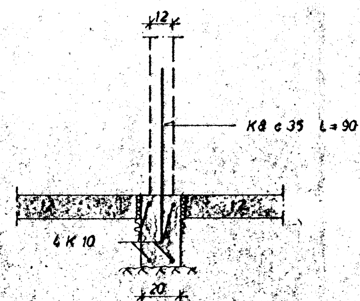
SNIÐ B 1:20
