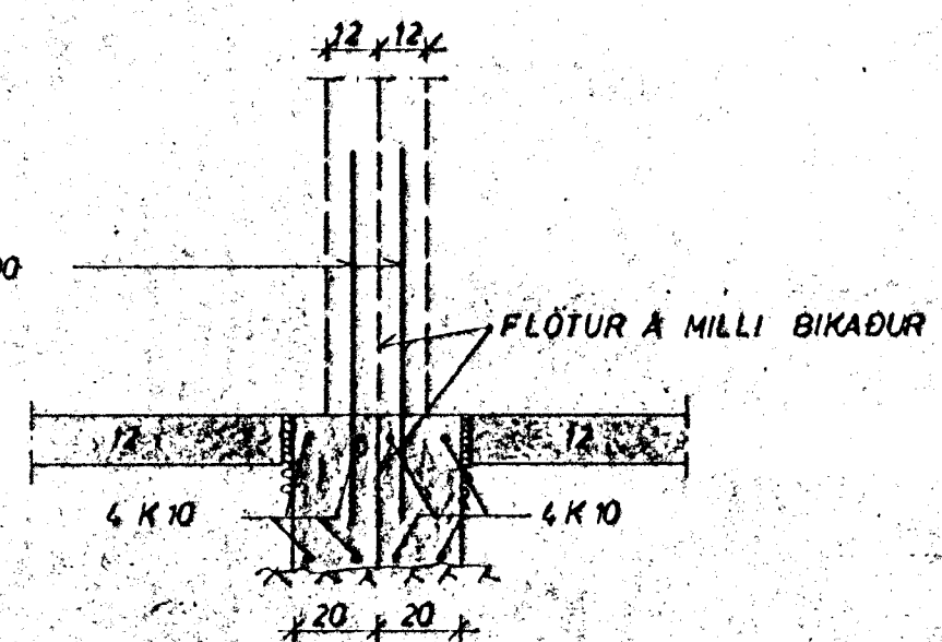
SNIÐ C 1:20
