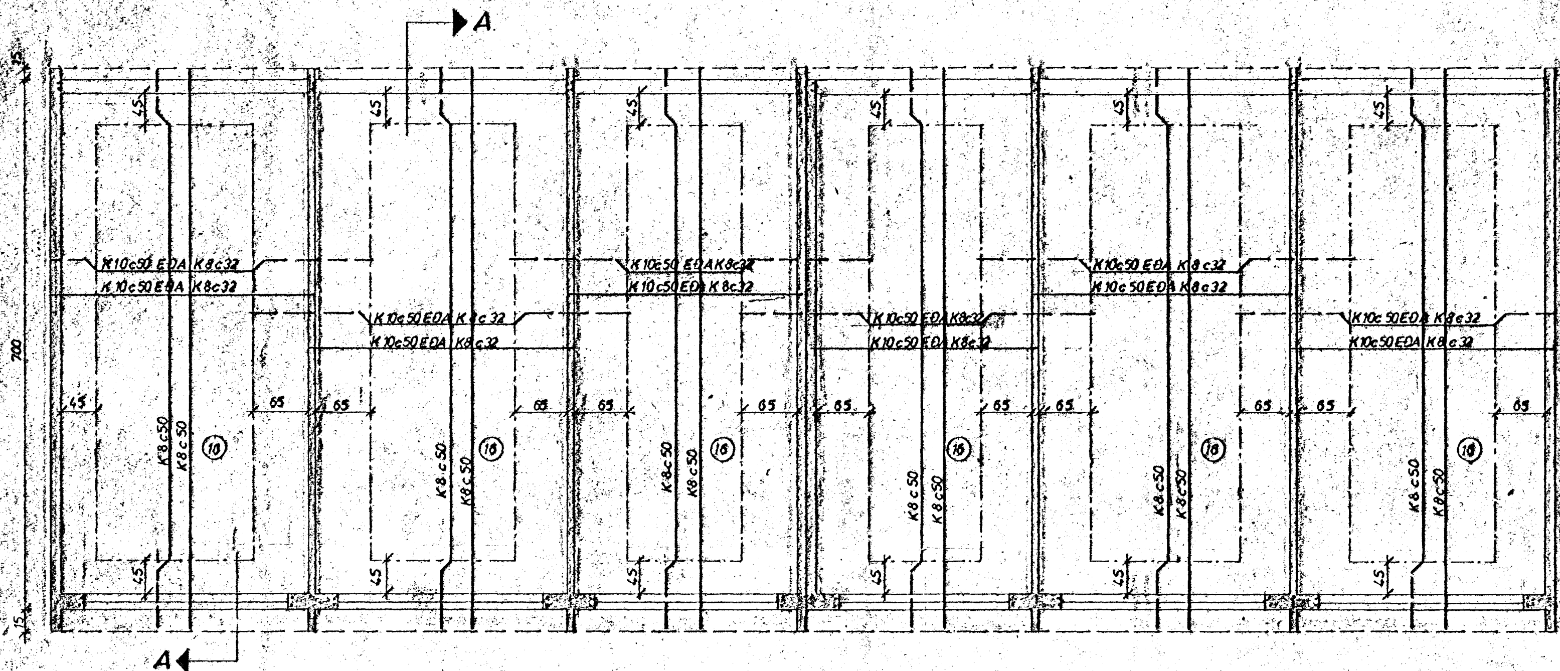
GRUNNMYND 1:50
