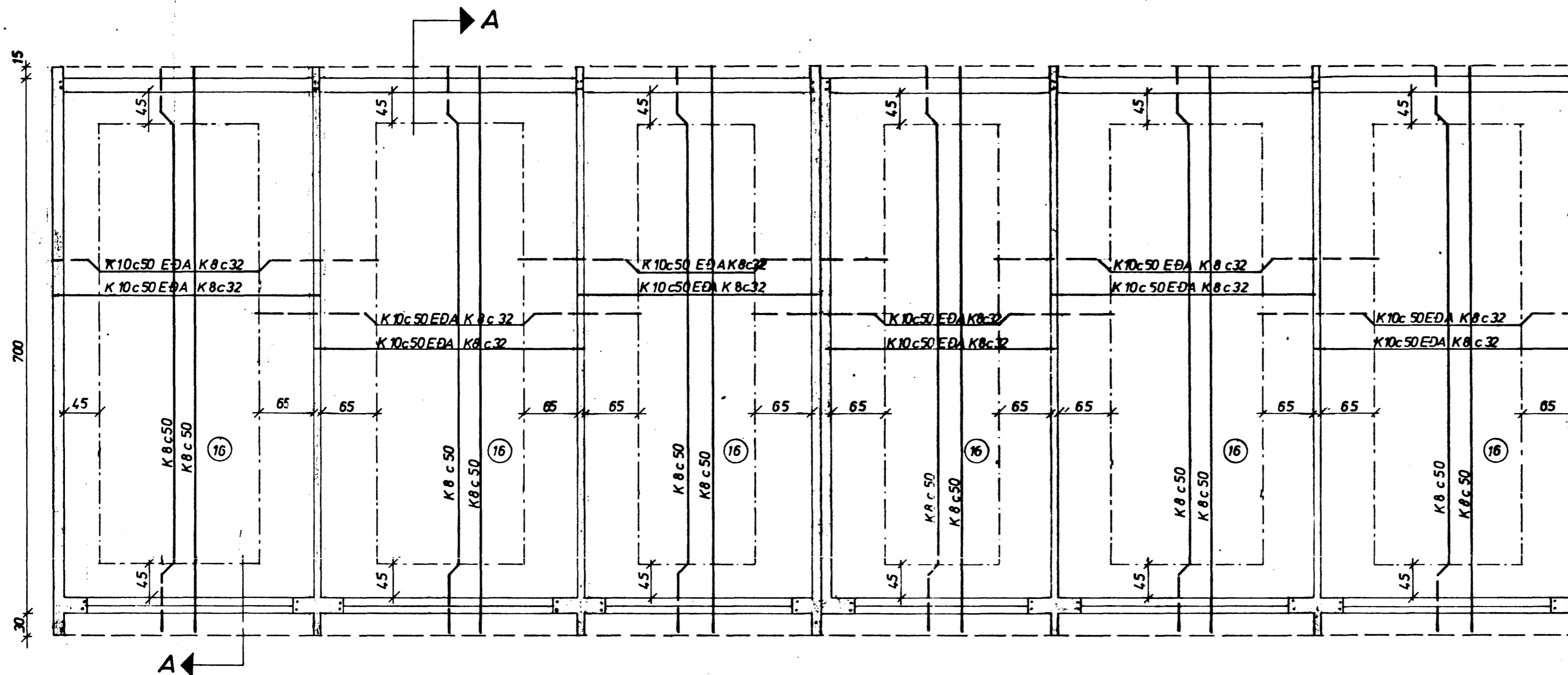
GRUNNMYND 1:50
