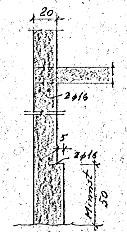
Snid A-A 1:20
