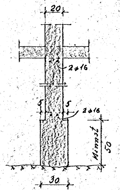
Snid D-D 1:20
