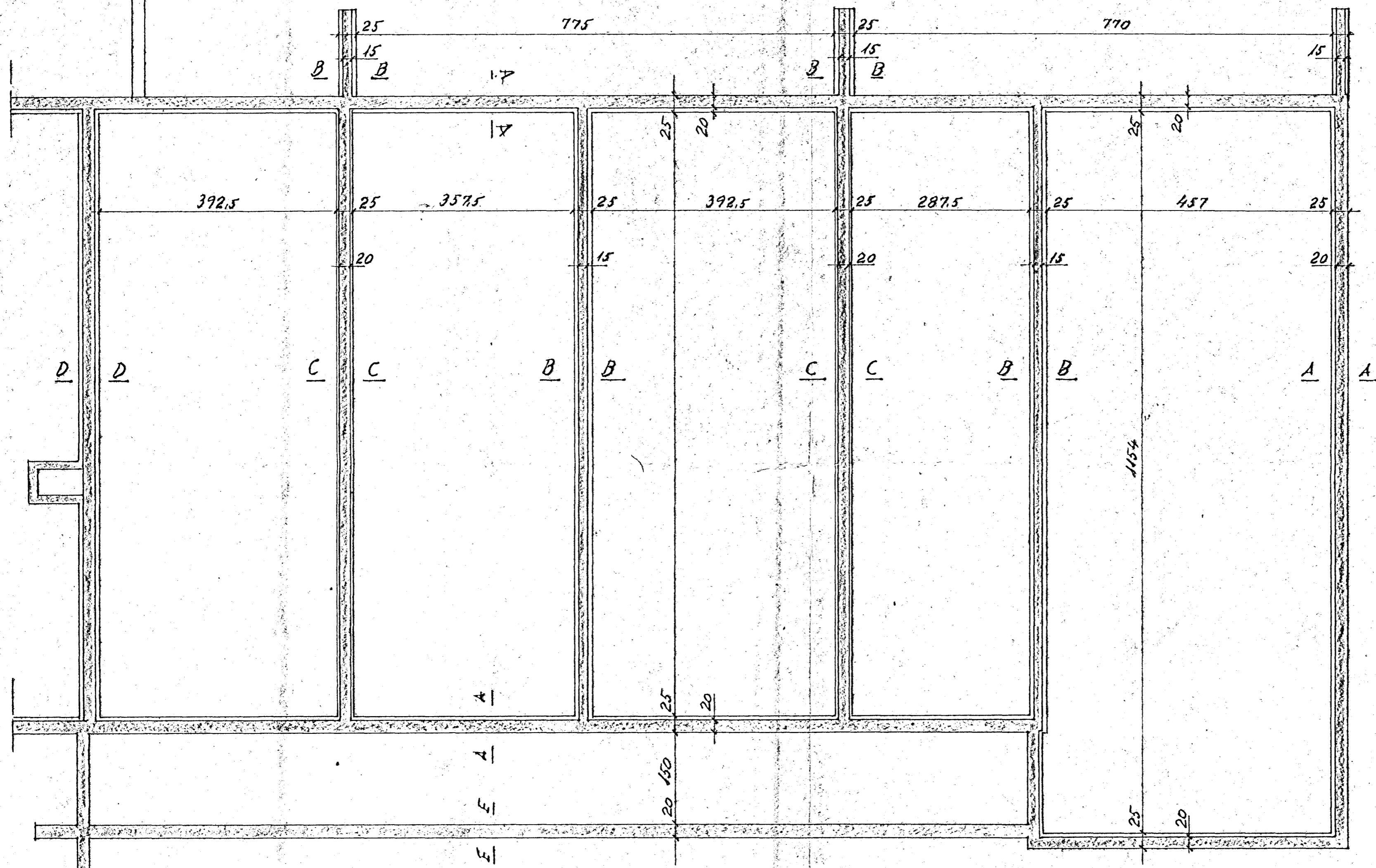
Grunnmynd 1:50
