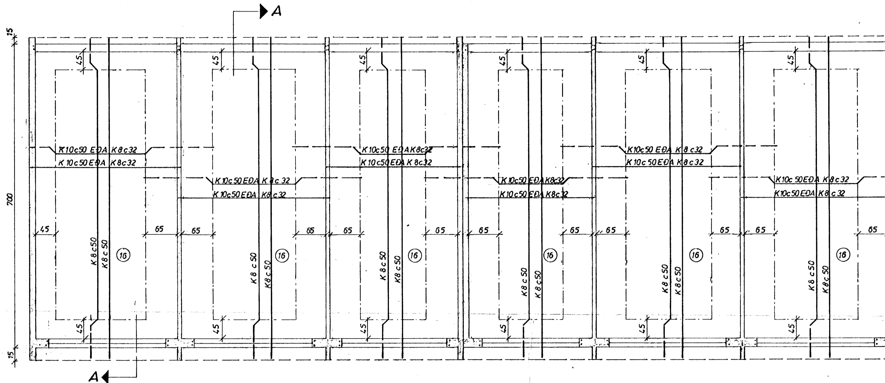
GRUNNMYND 1:50
