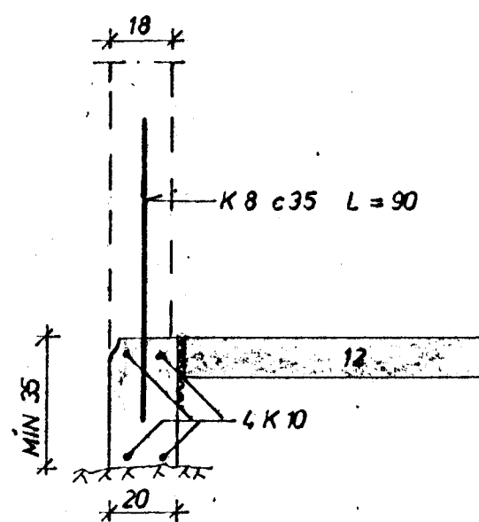
SNIÐ A 1:20
