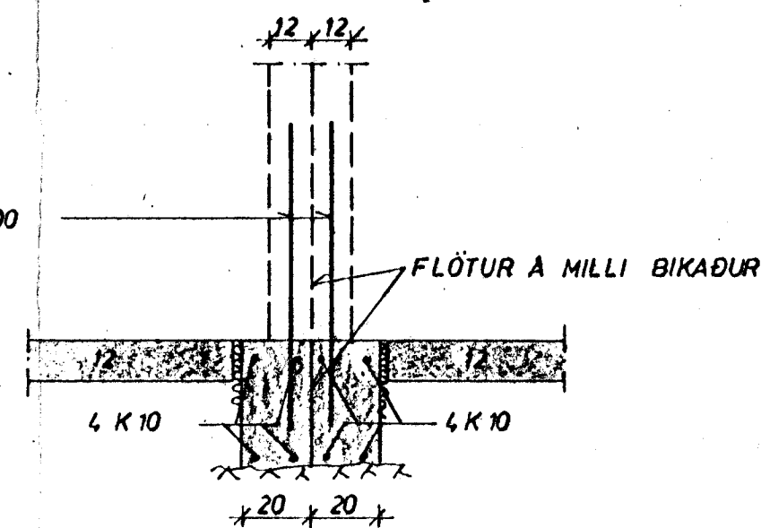
SNIÐ C 1:20
