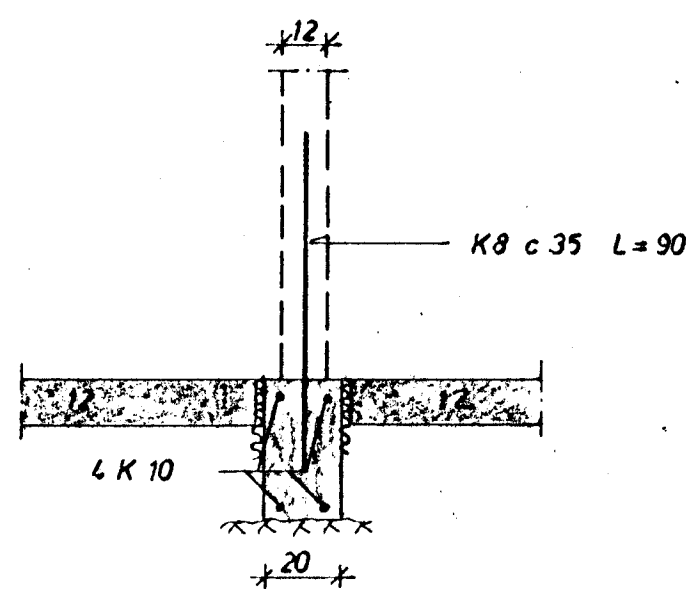
SNIÐ B 1:20
