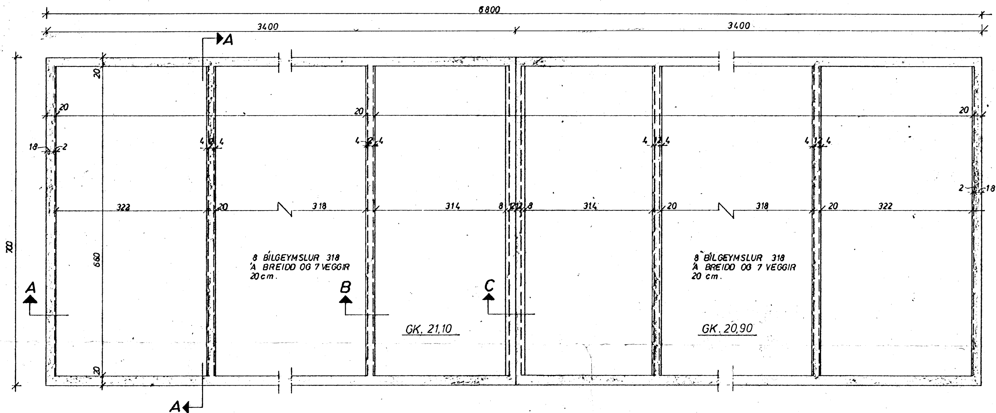
GRUNNMYND 1:50
