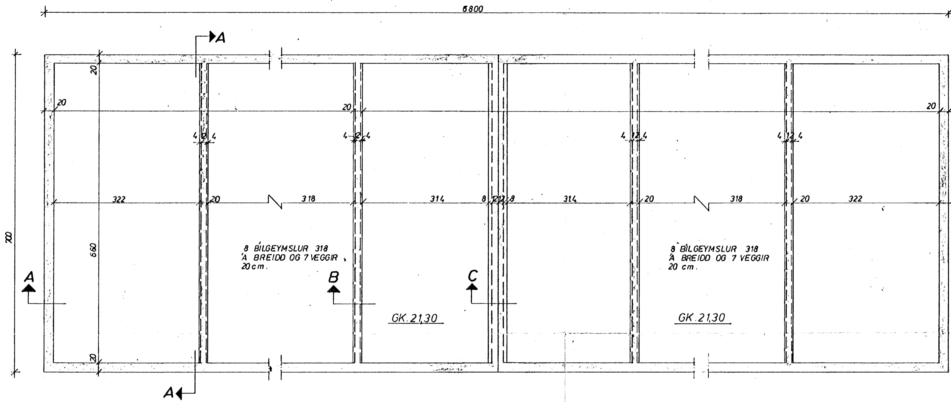
GRUNNMYND 1:50
