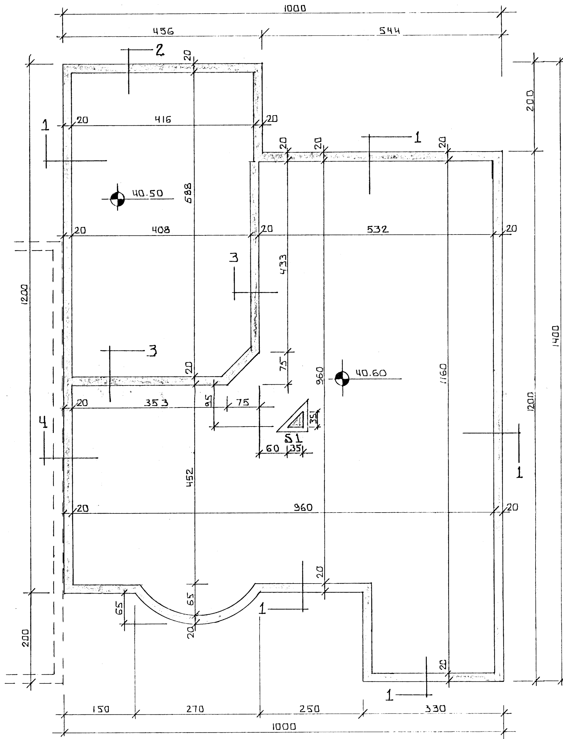
GRUNNMYND 1 HÆÐ 1:50
