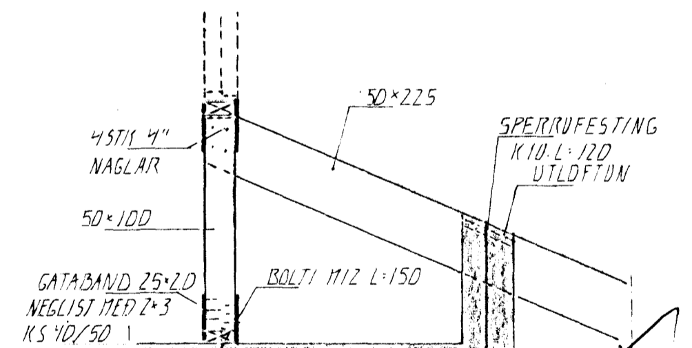
SNID A. 1:20
