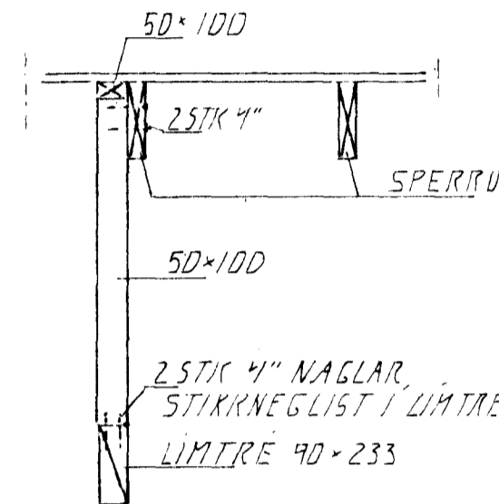
SNID 2. 1:20
