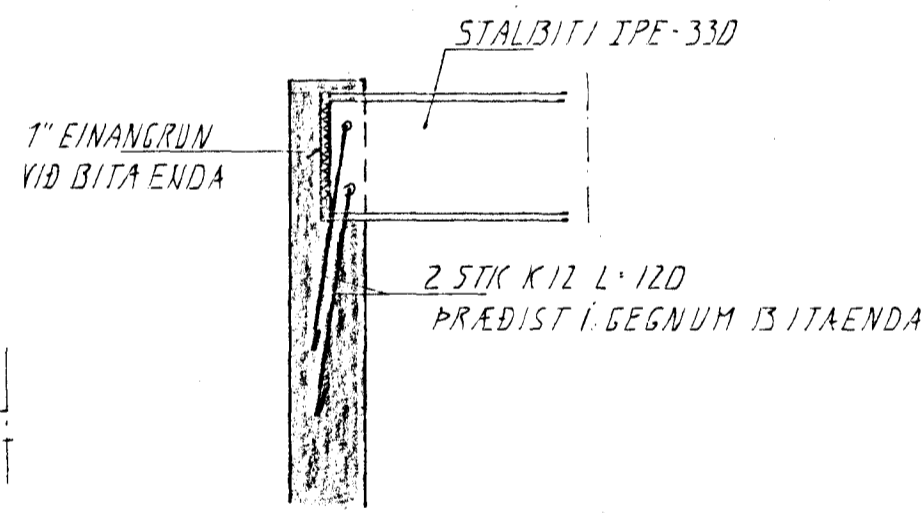
SNID 3. 1:20
