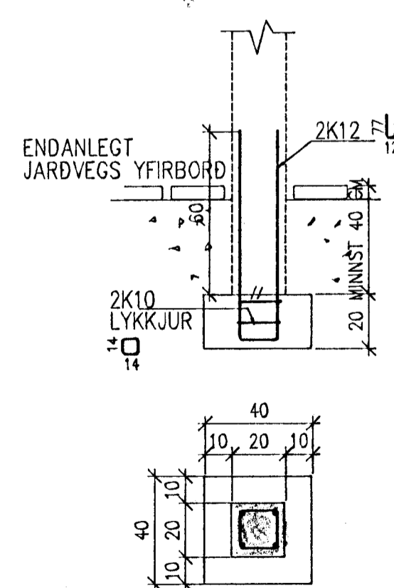
SÚLA UNDIR ÚTTRÖPPUM 1/20
