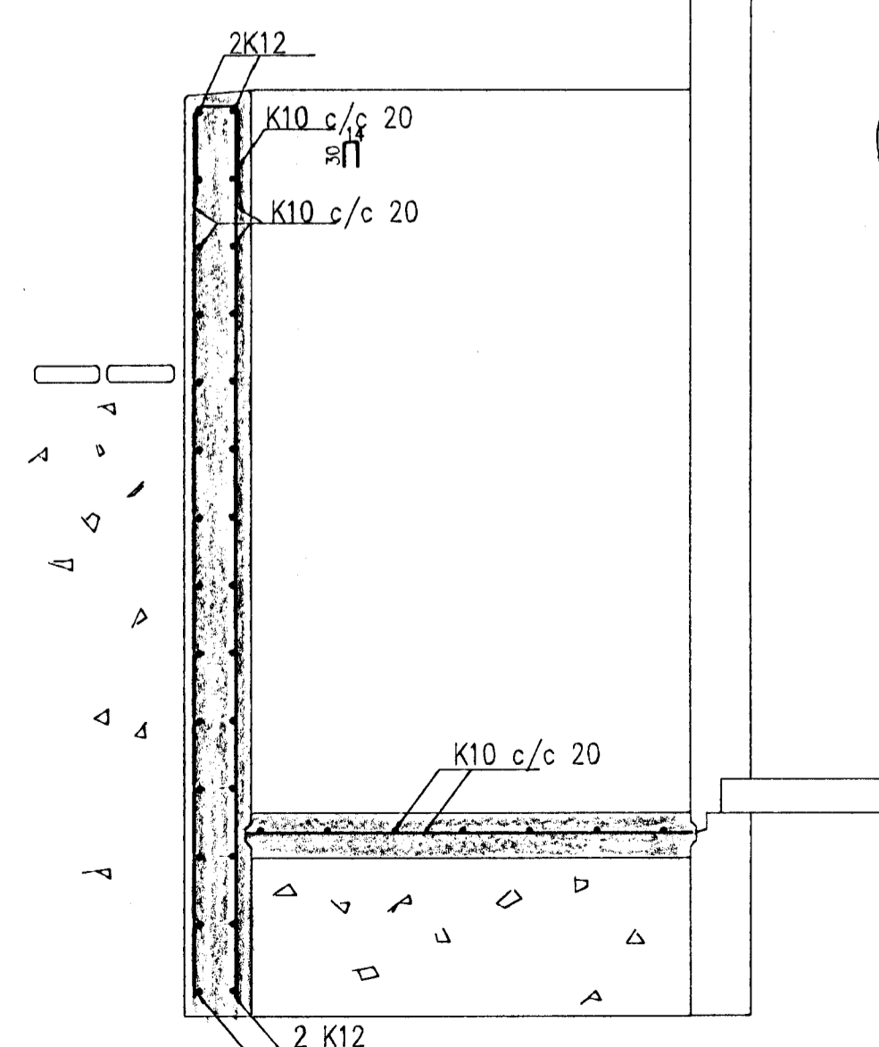
SNID Í VEGGI OG KJALLARATRÖPPUR
