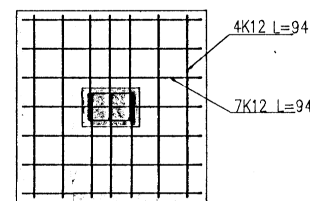
SÉÐ OFANÁ SÚLU S2
