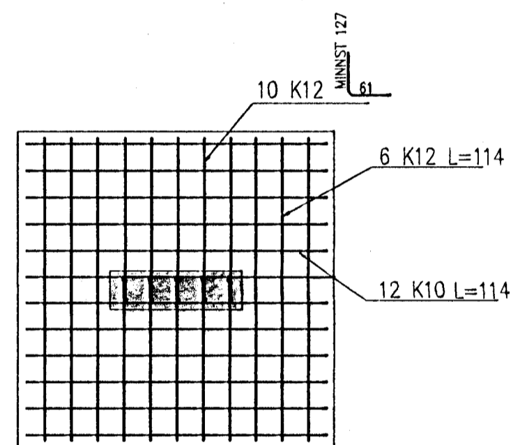
SÉÐ OFANÁ SÚLU S1
