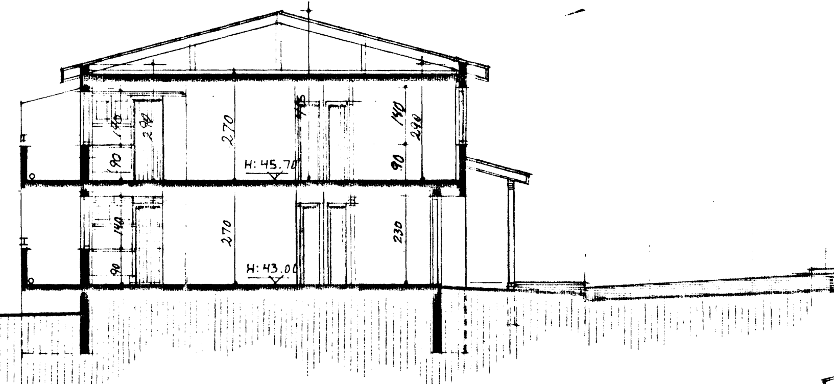
SNID A-A
