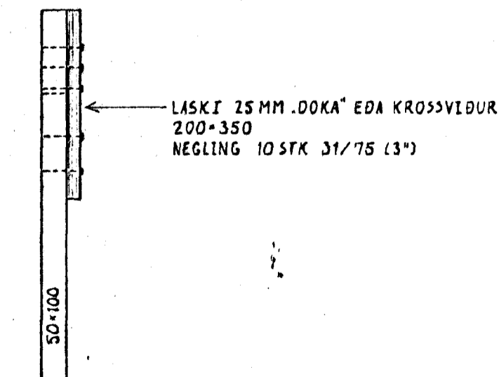
SNIÐ III a -III a 1:10 SÉRMYND III 1:10
