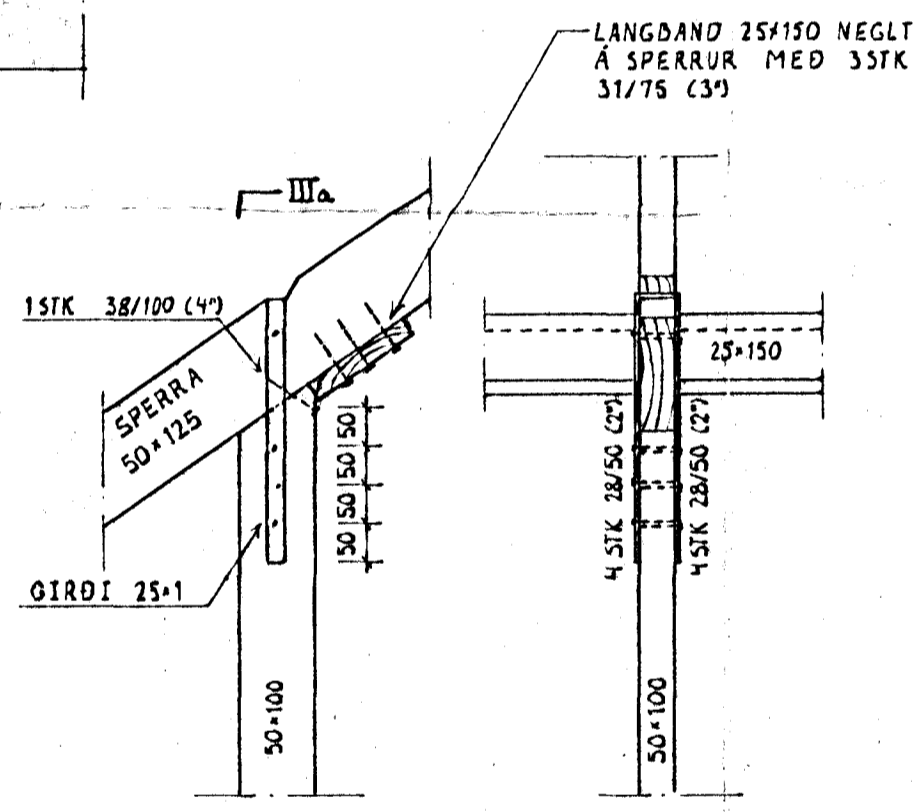
SNIÐ III a -III a 1:10 SÉRMYND III 1:10
