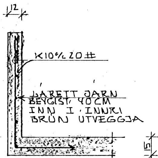
SNIB A-A 1:20
