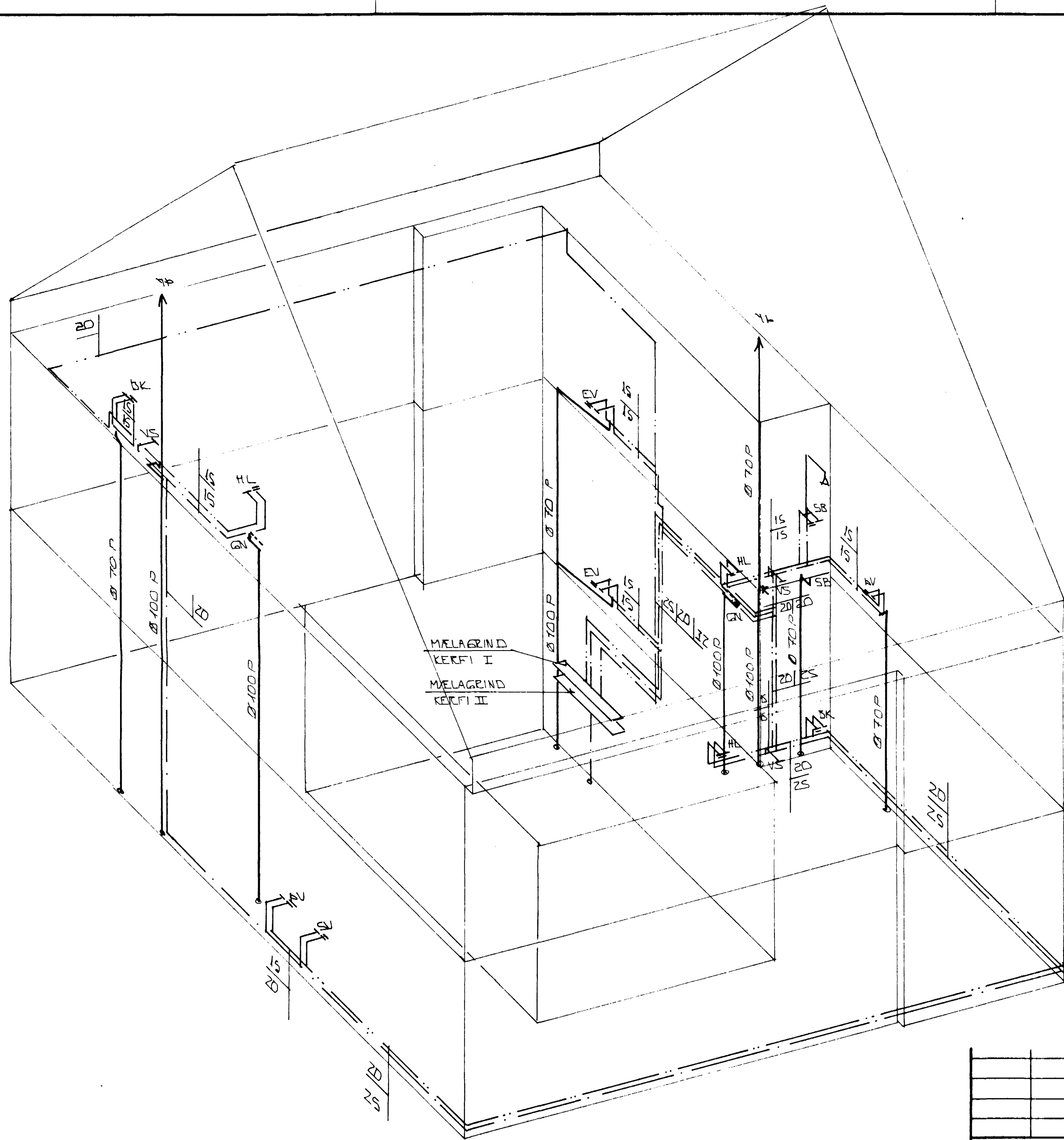
RÚMMYND VATNSLAGNA 1:50
