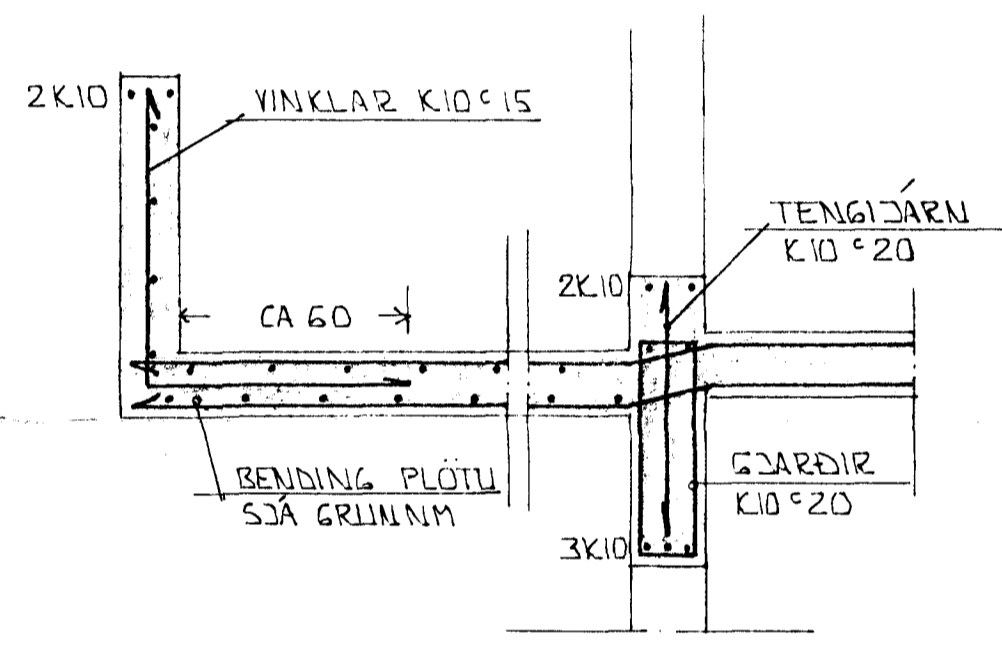
SNID 6-6 · 1 20
