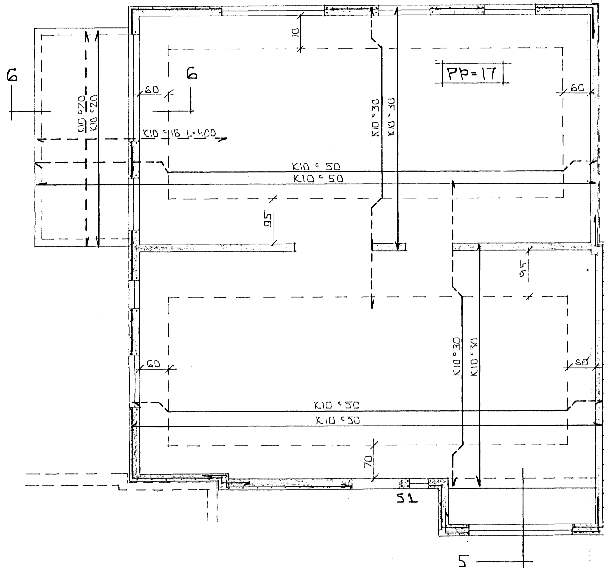
GRUNNMYND · 1 : 50
