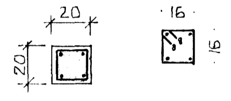
SÍLA S1 · 1 : 20
