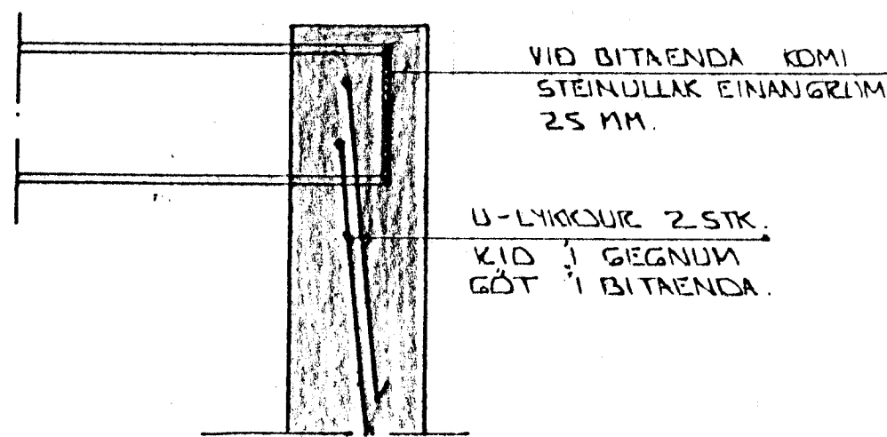
FRÁGANGUR STALBITA Í VEGG
