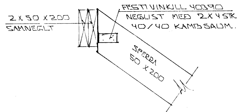
SNID G 1:20
