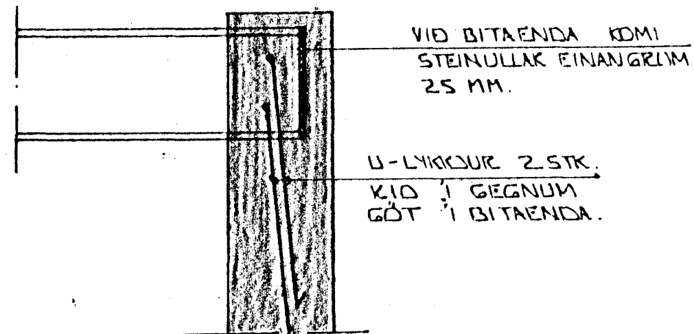
FRÁGANGUR STÁLBITA Í VEGG 1:10
