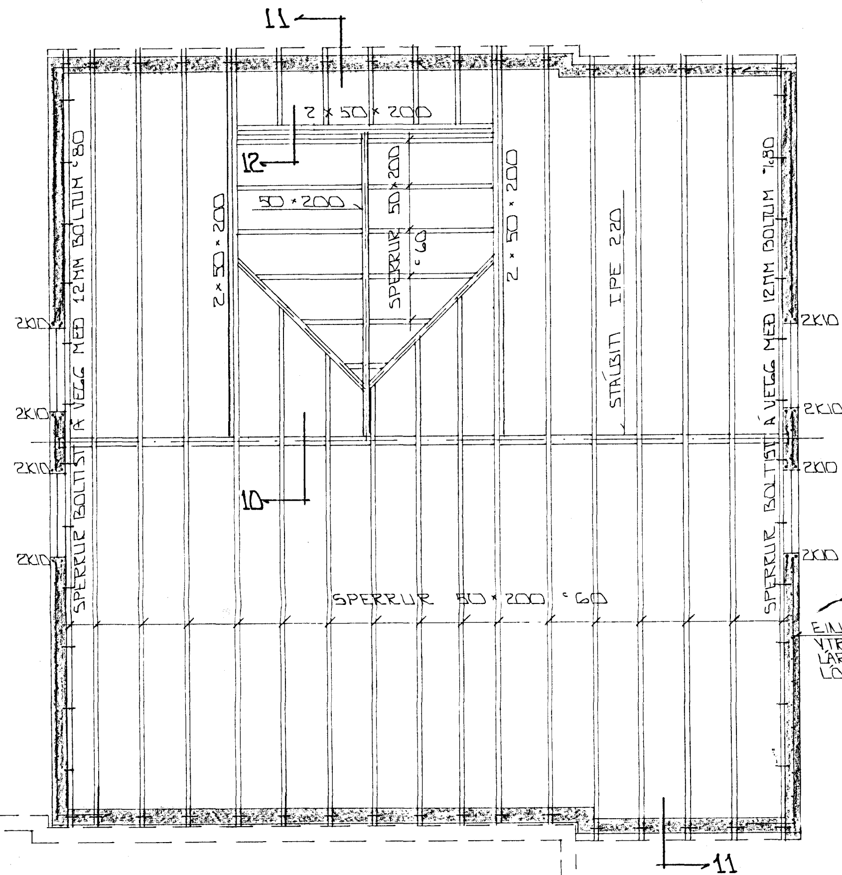
GRUNNMYND 1:50
