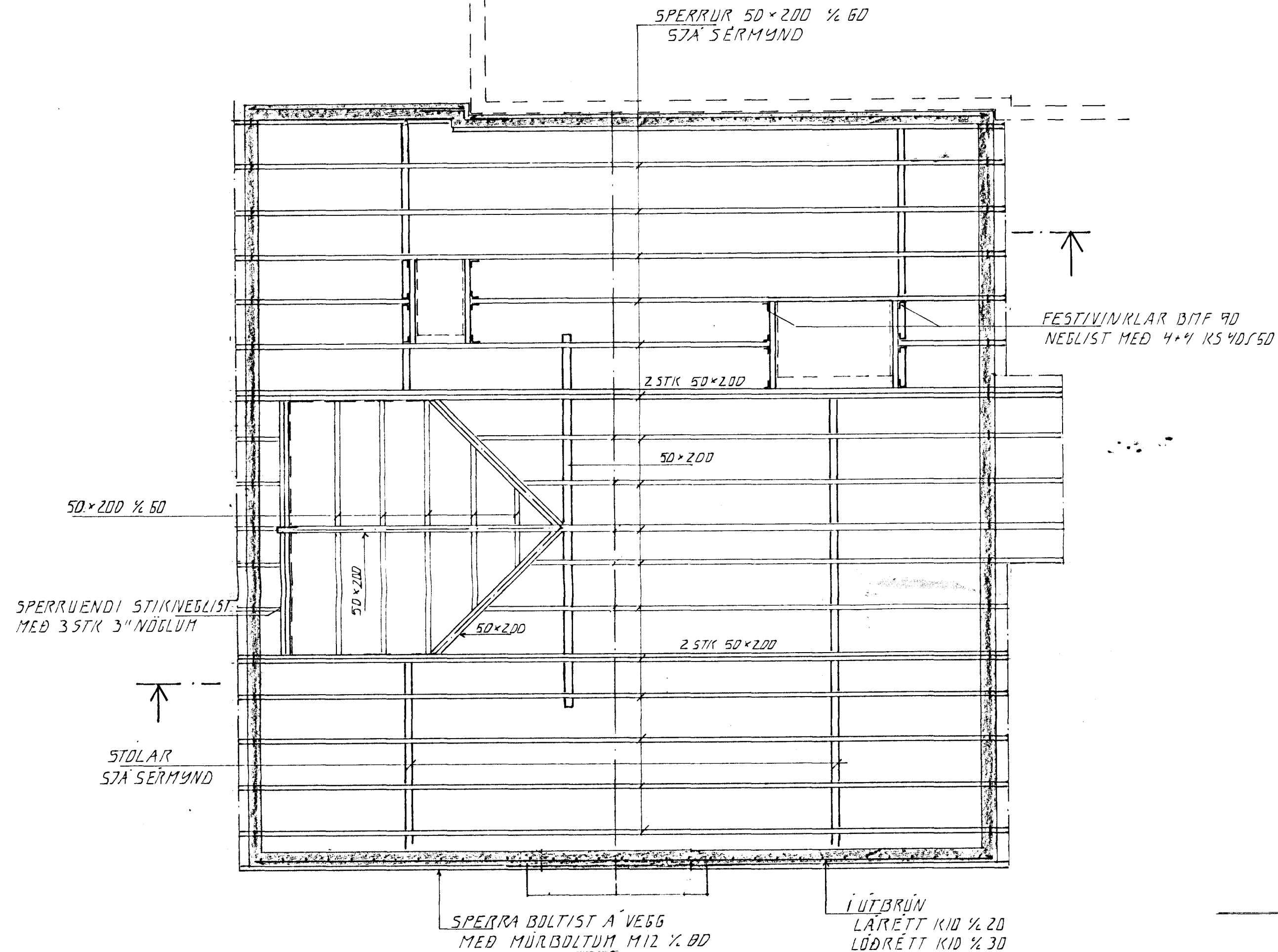
GRUNNMÝND 1:50
