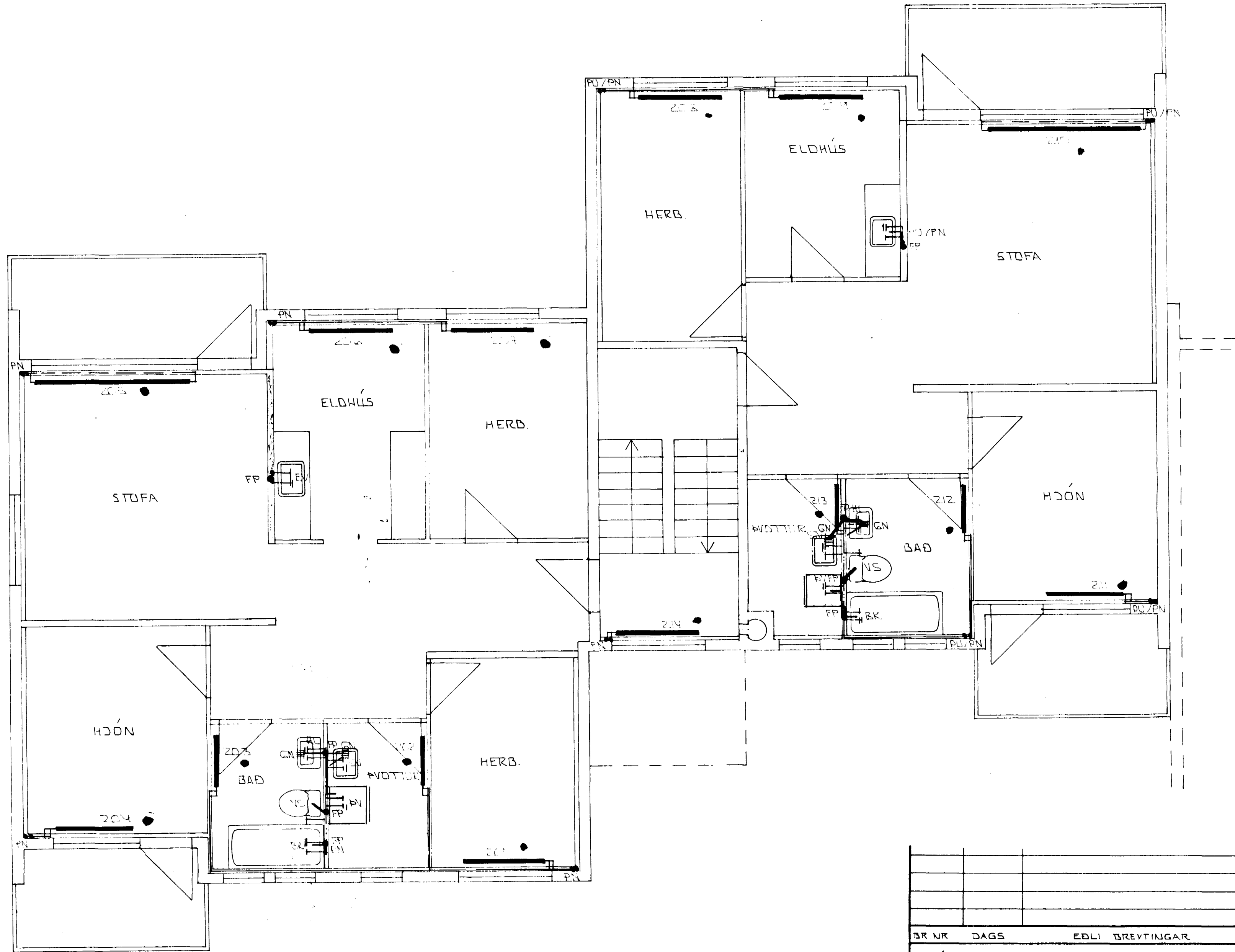
GRUNNMYND 2. HÆÐ 1:50
