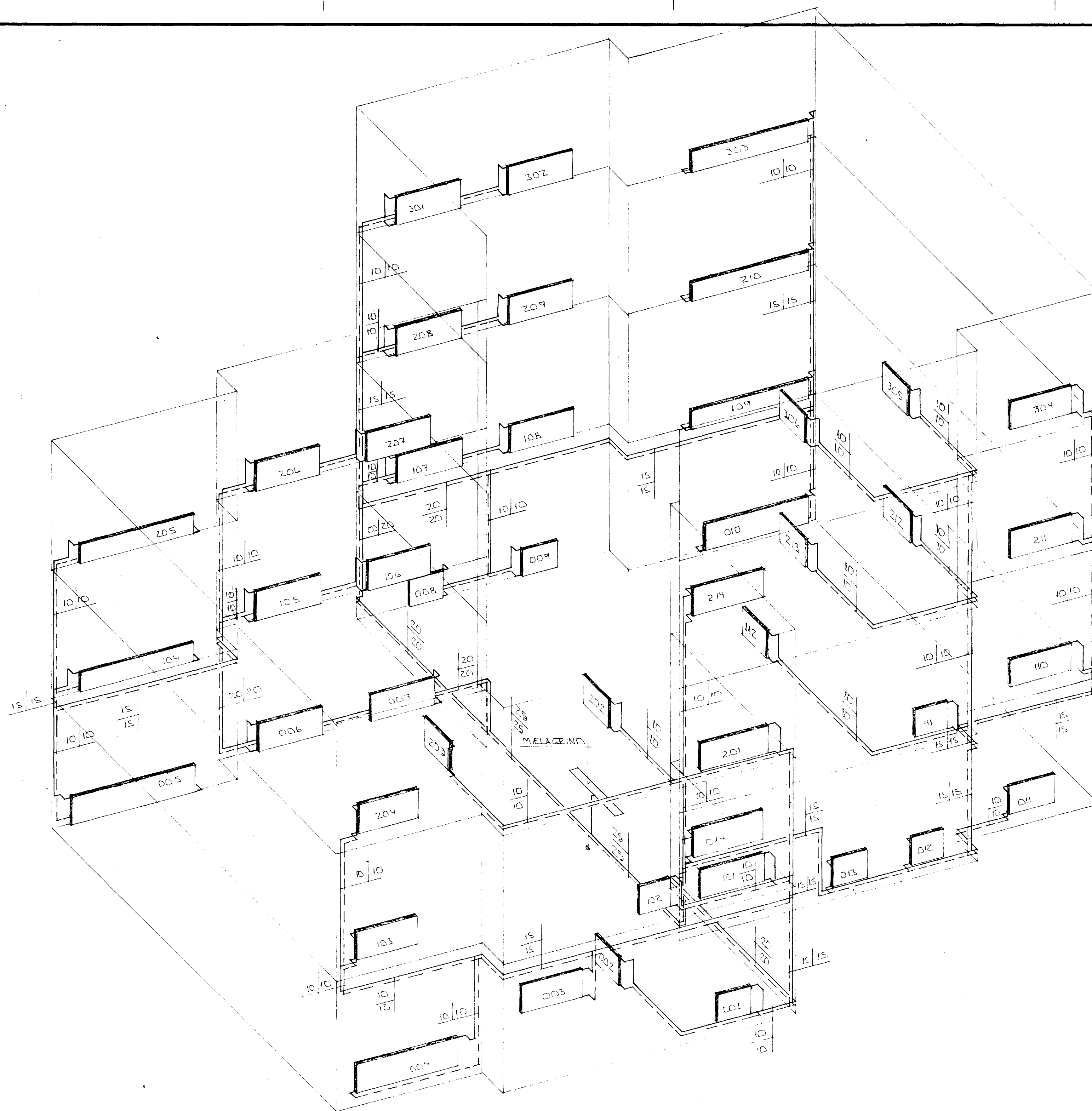
RÚMMYND HITLAGNA 1:50
