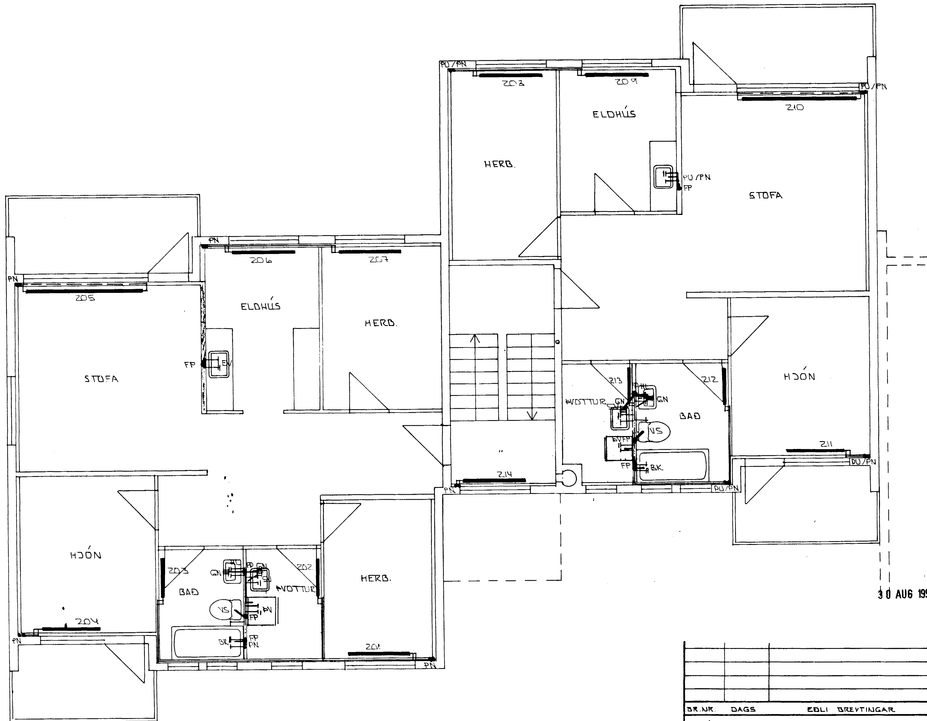
GRUNNMYND 2. HÆÐ 1:50
