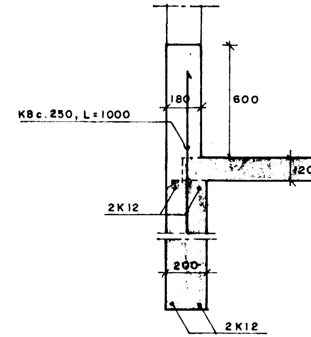
SNID D05 1:20
