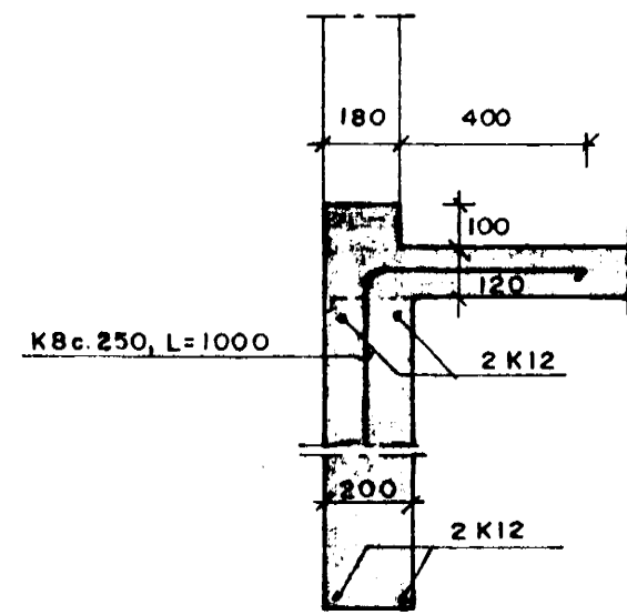
SNID E05 1:20
