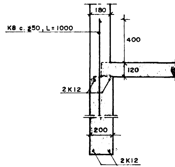
SNID A05 1:20
