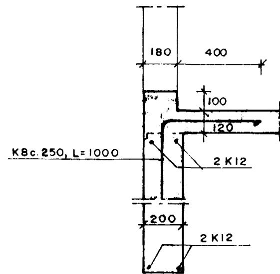
SNID E05 1:20
