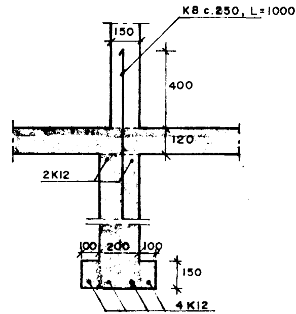
SNID C05 1:20
