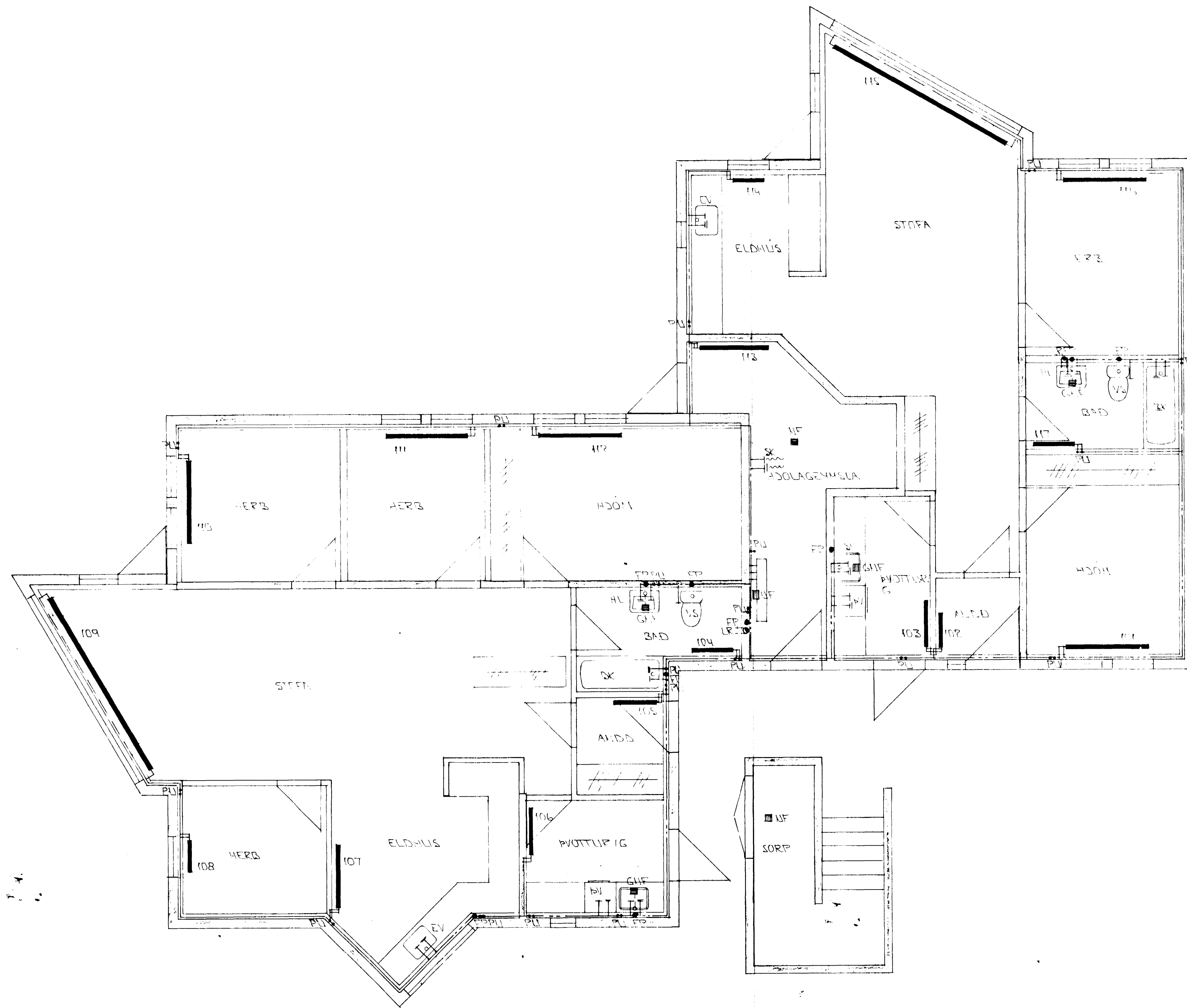
GRUNNMÝND 1. HÆÐAR 1:50
