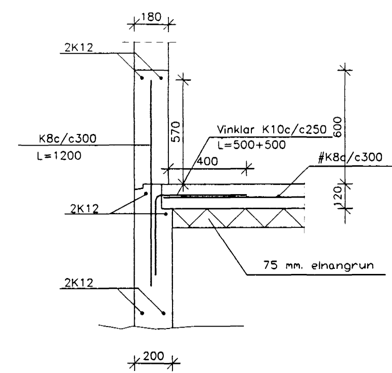
SNID D05 1:20
