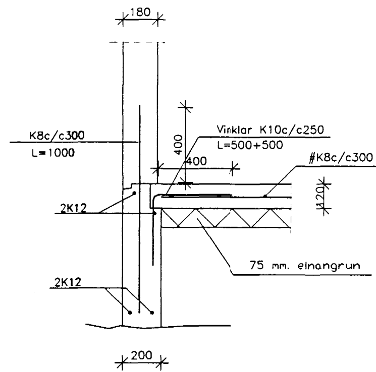
SNID A05 1:20
