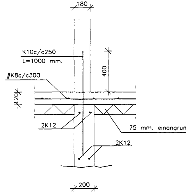
SNID C05 1:20
