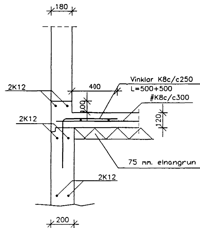
SNID E05 1:20
