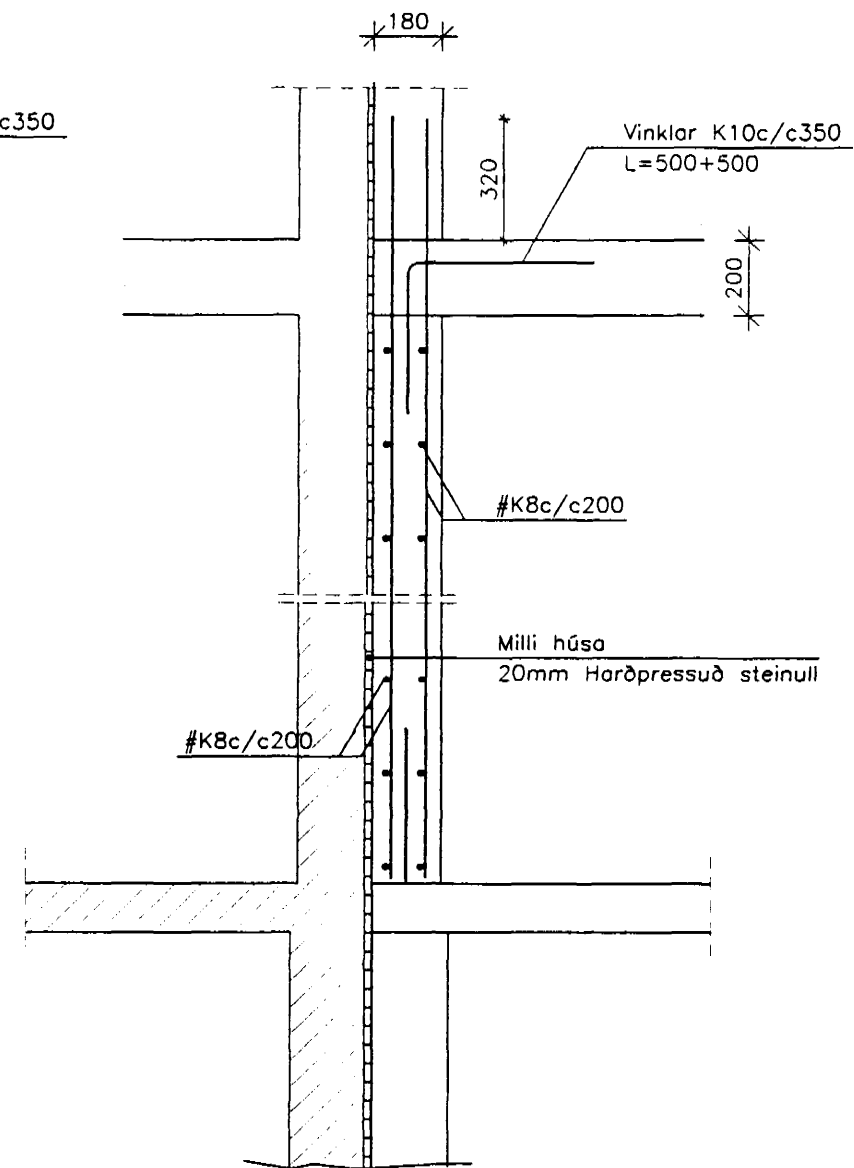
SNID D07 1:20
