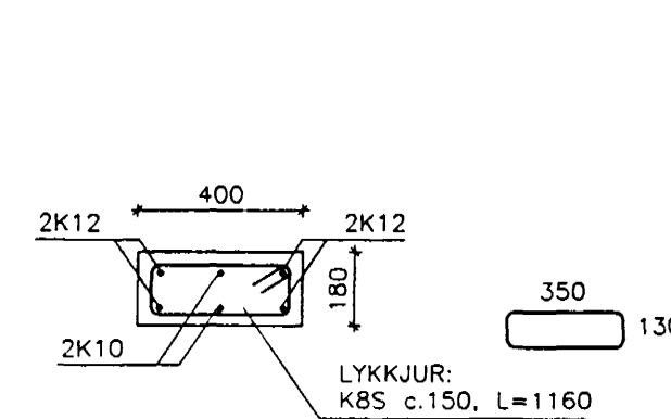
SÚLA S3-06 1:20
