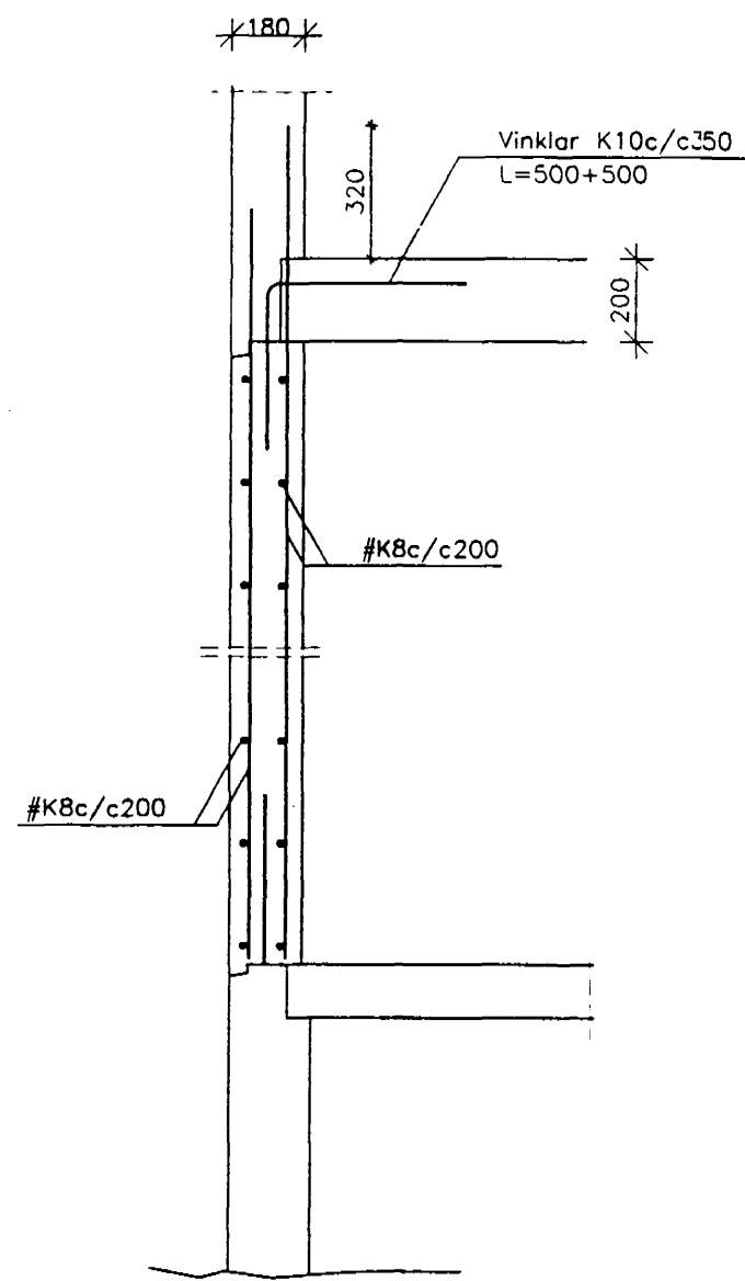
SNID A07 1:20
