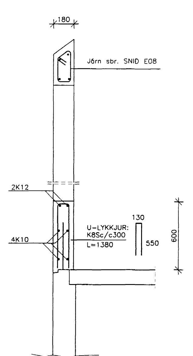
SNID E07 1:20
