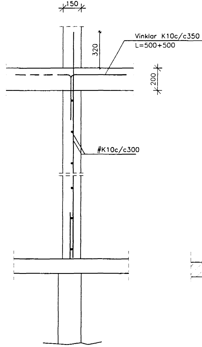
SNID C07 1:20
