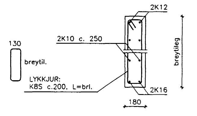
SNID H07 1:20
