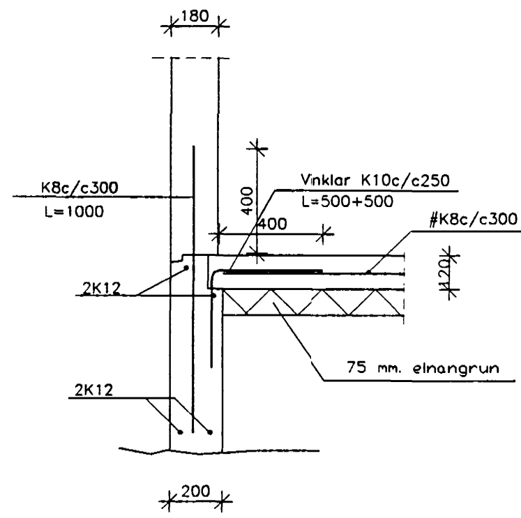
SNID A05 1:20
