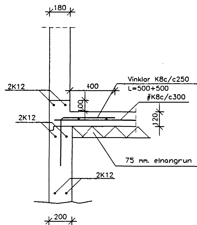
SNID E05 1:20
