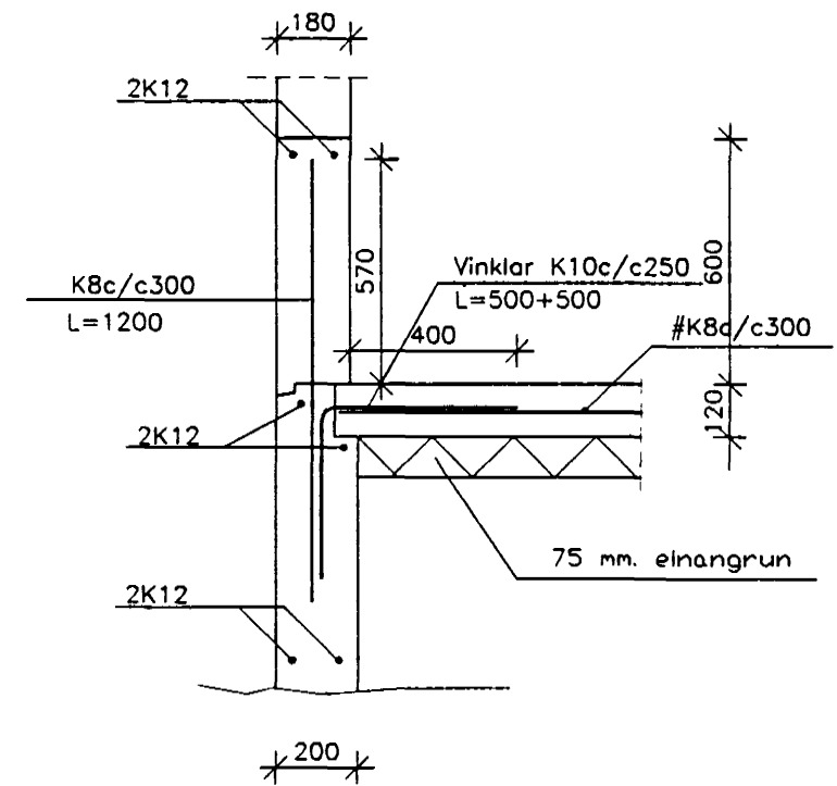
SNID D05 1:20
