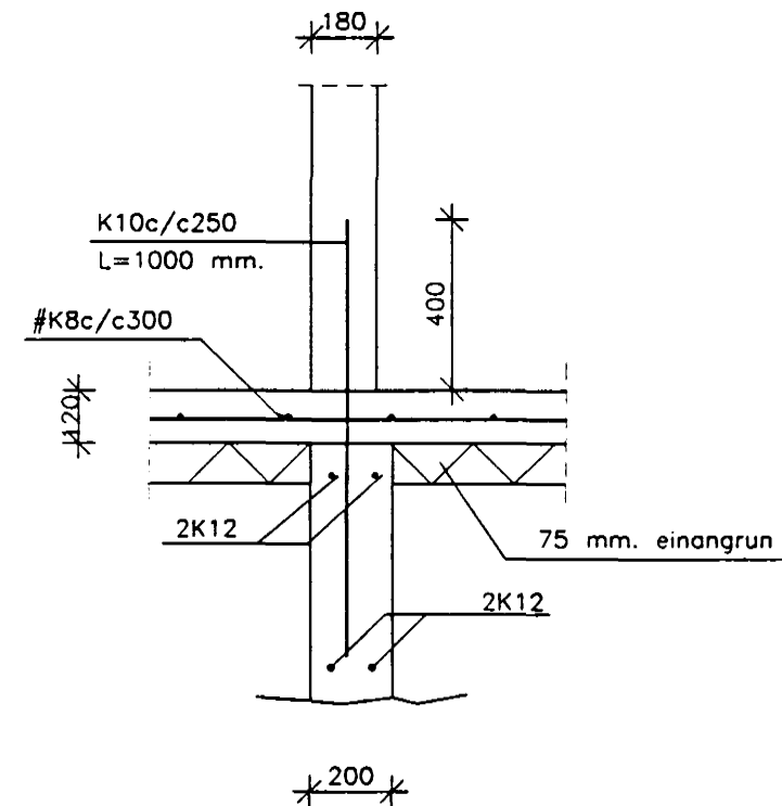
SNID C05 1:20
